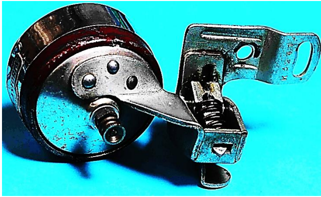
Bild 12.31: Kippschalterprinzip: a) Boden mit Kabelanschlussbolzen und angenietetem Flansch der Kippvorrichtung, b) Kippvorrichtung mit der K-Nummer K 32412
