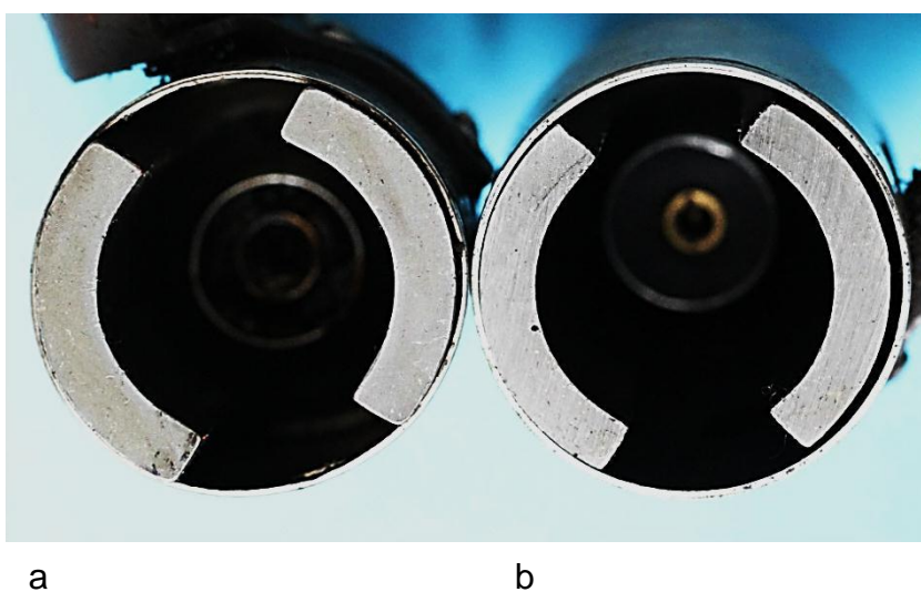
Bild 6.10: Stirnflächen der Magnetpole: a) Impex-Saba, 7 mm dick, 60 mm lang b) Impex-Super, 6 mm dick, 65mm lang
