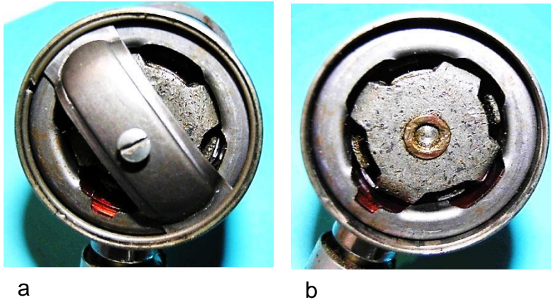
Bild 12.35: Abgenommener Boden: a) Steg mit Bodenschraube, b) Stirnseiten des Polrades und des Ankers
