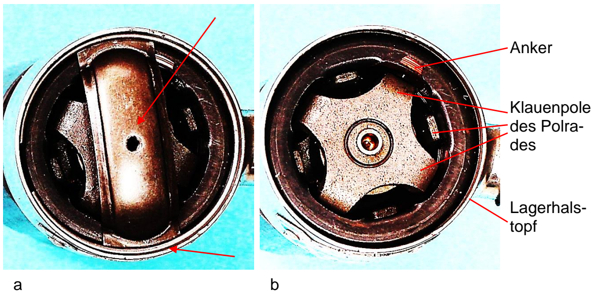
Bild 12.41: Generator mit Klauenpolen im Anker und im Polrad: a) Spannstege zur Bodenbefestigung und Drahtfeder zur axialen Sicherung des Ankers, b) Stirnseiten des Polrads und des Ankers:
