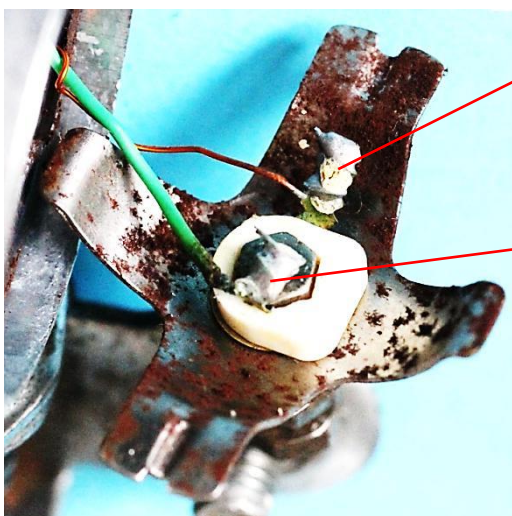
Bild 12.68: Kontakte am Montagegesteg für beide Spulenenden
