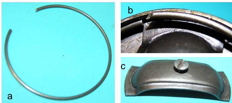
Bild 12.36: Montageteile a) Drahtfeder b) Eingelegter Drahtfeder- ring c) Montagesteg
