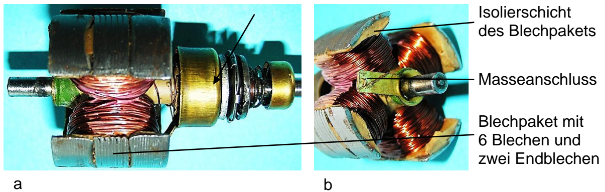
Bild 11.10: Ankeranschlüsse: a) Spannung führender Kontakt, b) Lötfläche für den Massekontakt
