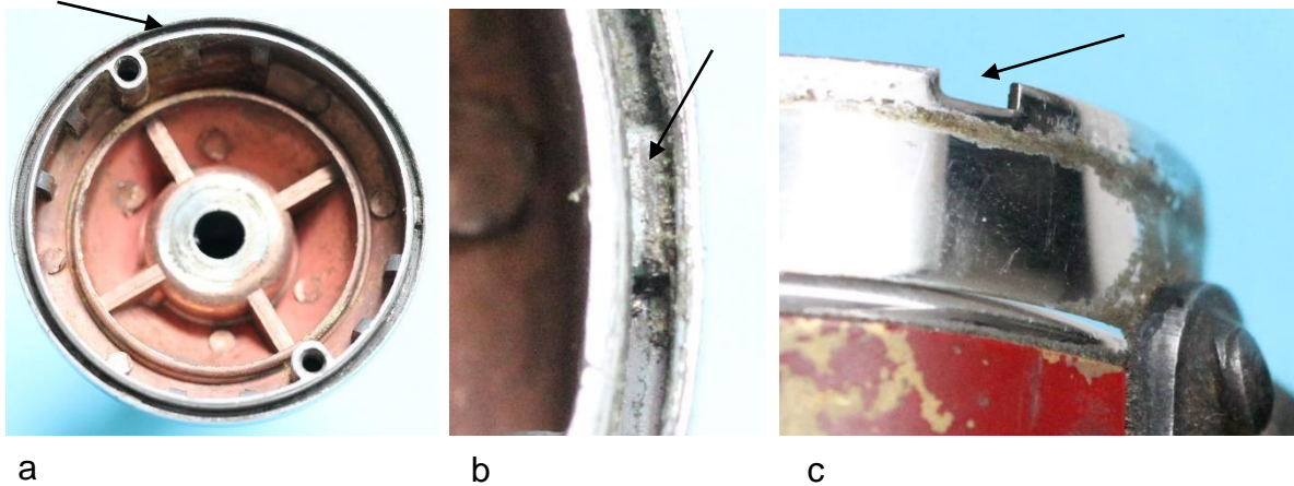
Bild 12.2: Wasserdichte Einpassung des Gehäusetopfes im Lagerhalsfuß: a) 2 mm tiefe Rille im Lagerhalsfuß, b) Zapfen in der Rille, c) Ausnehmung im Gehäuserand
