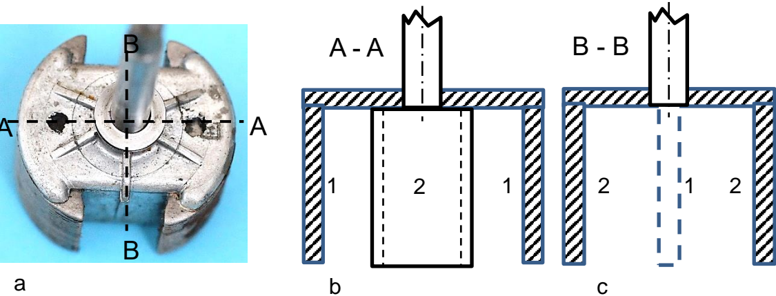
Bild 12.20: Polrad: a) Schnittebenen, b) Schnitt A-A, c) Schnitt B-B, 1-Polstab, 2-Pollückensteg
