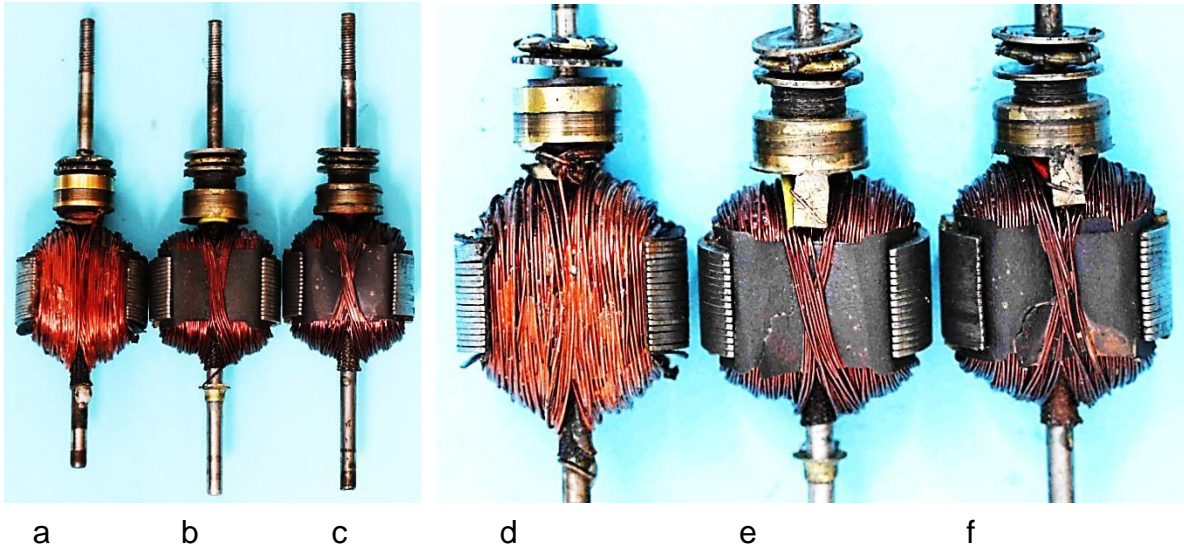
Bild 6.21: Anker: a) Impex-Saba, b) Impex-Super, c) Impex 30, d) Impex-Saba, e) Impex-Super, f) Impex 30,
