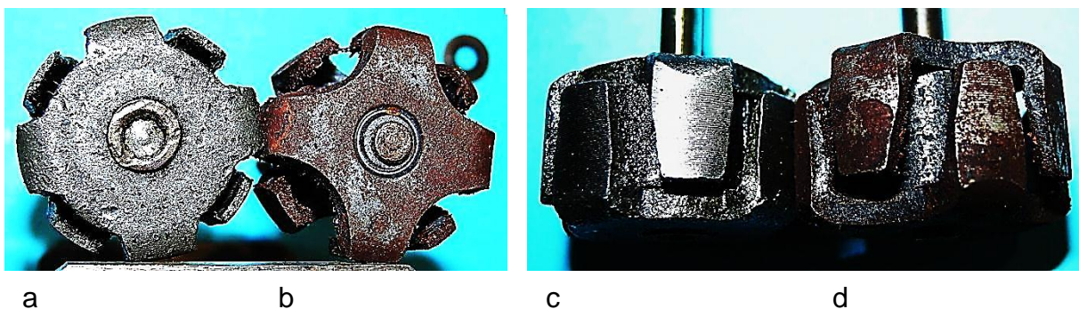
Bild 12.46: Gegenüberstellung ausgewählter Polräder
