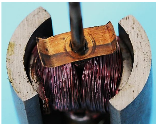
Bild 9.22: Massekontakt: a) Kontaktfeder mit zwei Kontaktstellen, b) Schleifring
