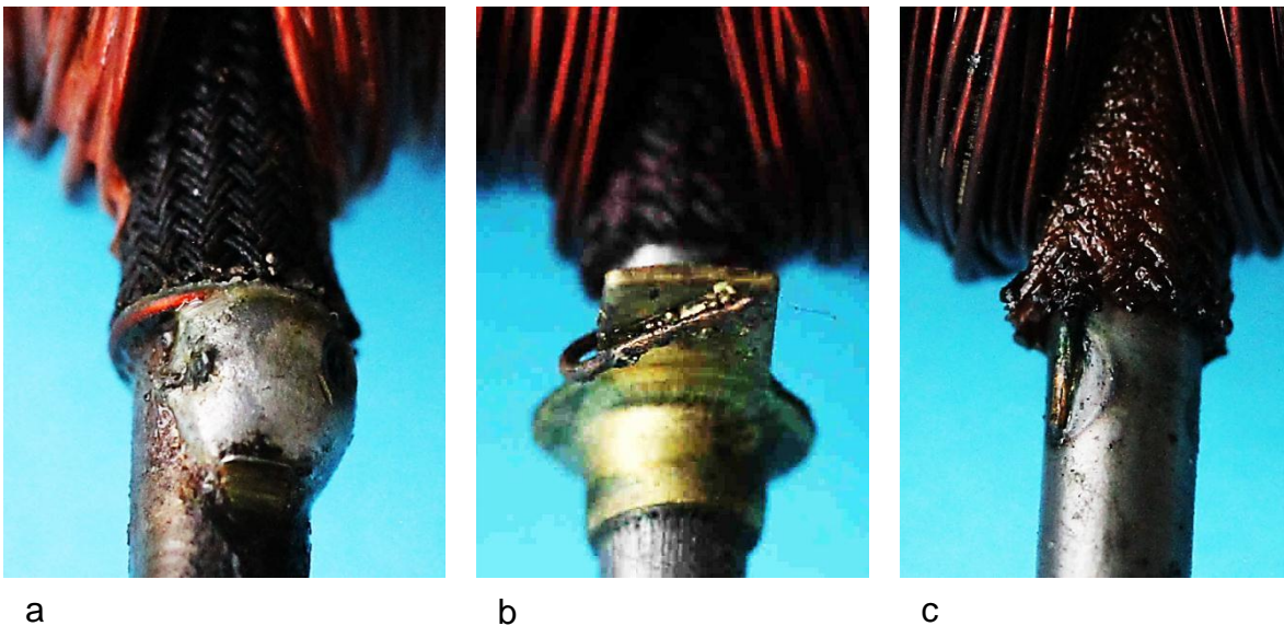
Bild 6.20: Massekontakte: a) Impex-Saba, b) Impex-Super, c) Impex 30
