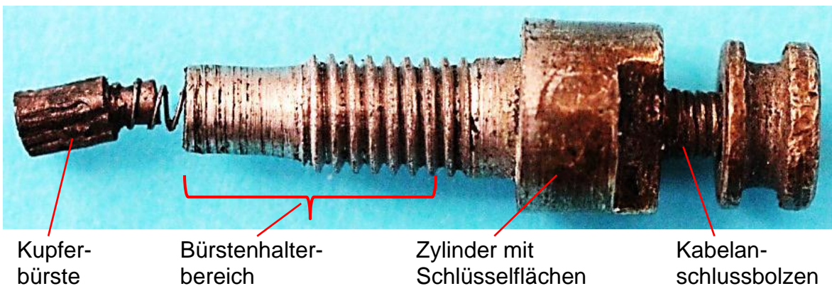
Bild 7.10: Kombination aus Bürstenhalter und Kabelanschlussbolzen
