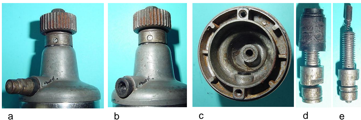
Bild 7.20: Position des Bürstenhalters im Lagerhalsfuß: a) Lagerhals mit Kabelanschluss, b) Entfernter Kabelanschluss, c) Innenraum des Lagerhalses, d) Kabelanschluss mit Isolierteil zum Lagerhals, e) Kabelanschluss mit Bürste
