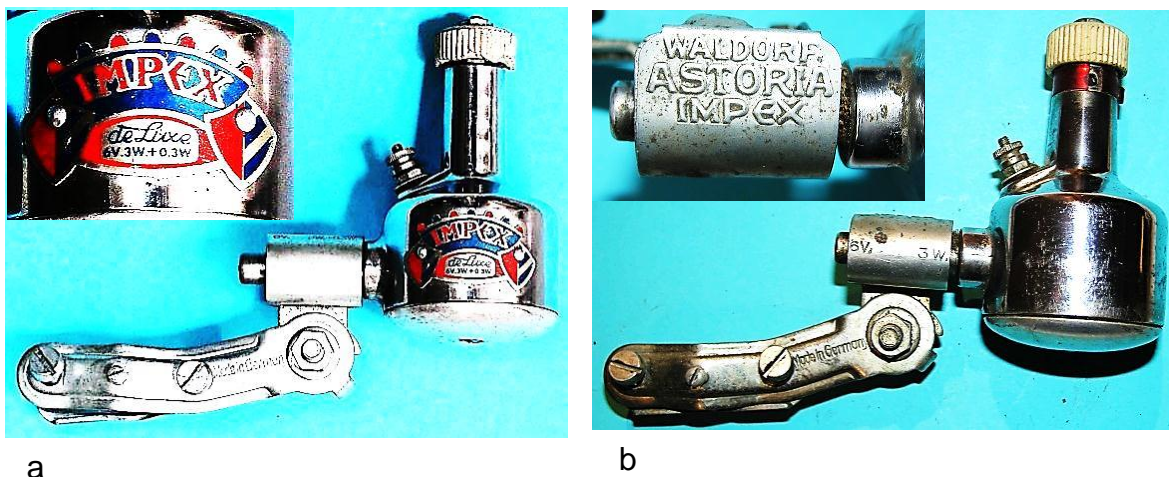
Bild 12.39: Gegenüberstellung ähnlicher Ausführungen: a) Impex de Luxe, b) Impex Astoria
