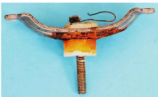
Bild 12.59: Zweiarmiger Montagegesteg
