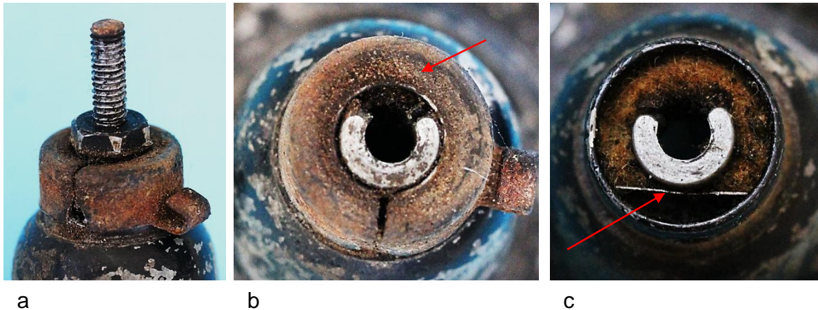
Bild 10.28: Öldepot: a) Abschluss des Lagerhalses, b) Drehbare Verschlusskappe, c) Ölfilz unter der Verschlusskappe mit Blech zum Freihalten der Ölbohrung (Pfeil)
