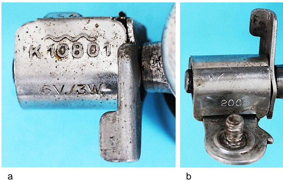
Bild 12.61: Einprägungen auf dem Abdeckblech
