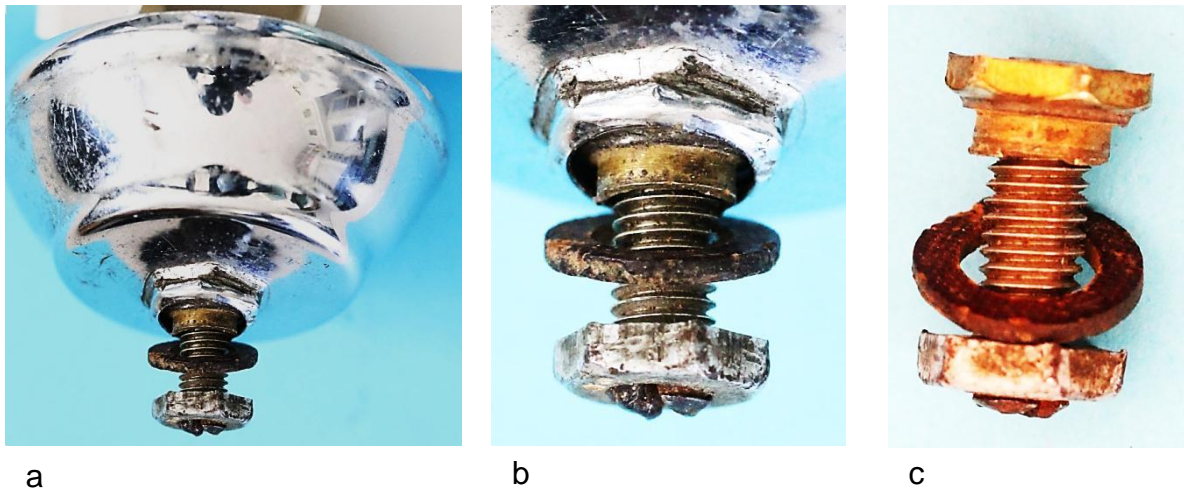
Bild 9.14: Bodenverspannung: a) Boden und Spannschraube, b) Verdrehsichere Positionierung der der Druckmutter im Boden, c) Spannschraube mit Druckmutter und Kontermutter
