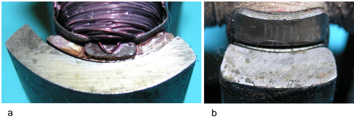
Bild 10.10: Unterschiede in der Polüberdeckung: a) 2-polige Variante: Ankerpollänge kürzer als die des Magneten, b) 4-polige Variante: Ankerpol- und Magnetpollängen sind identisch
