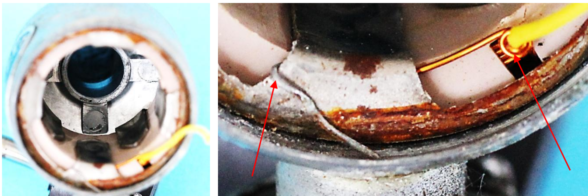
Bild 12.77: Spulenanschlüsse: a) Innenraum des Klauenpolankers, b) Masseanschluss und isoliertes Spannung führende Wicklungsende
