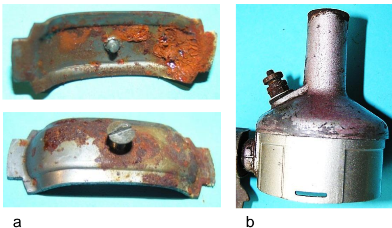
Bild 12.43: Lagerhalstopf: a) Montagesteg, b) Lagerhalstopf mit Schlitz für das Einklinken des Montagestegs
