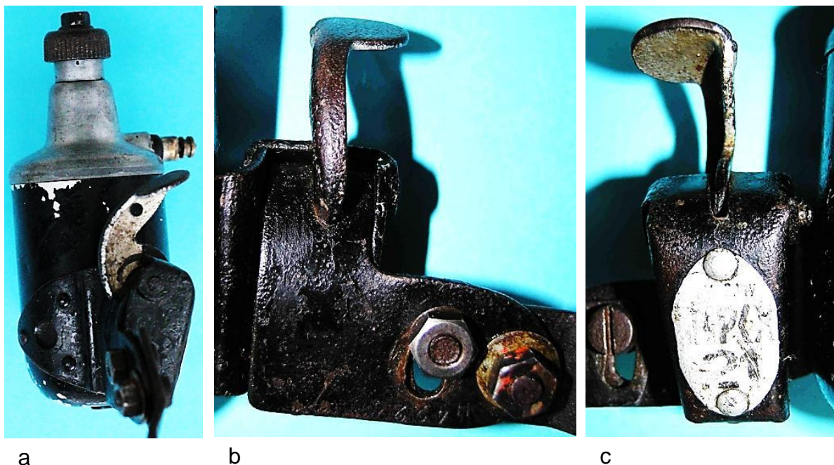
Bild 7.7: Kippvorrichtung: a) Schmalseite der Kippvorrichtung, b) Halterarm, c) Basisblech mit Firmenschild
