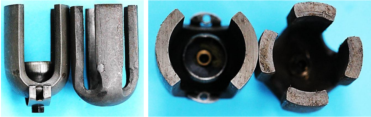
Bild 10.30: Zwei- und vierpolige Tulpenmagnete: a) Seitenansicht, b) Stirnseiten der Pole
