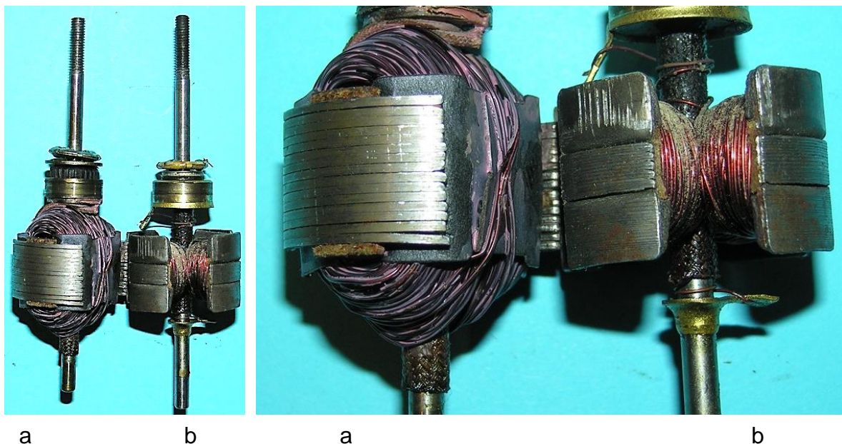
Bild 10.8: Gegenüberstellung eines Doppel-T-Ankers mit einem Sternanker mit gleichen Durchmessern
