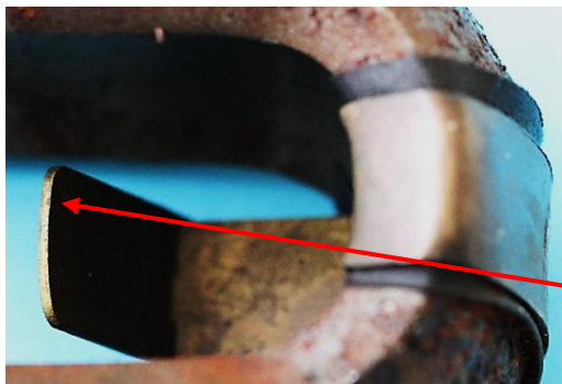
Bild 9.31: Kontaktblechbasis: a) Isolierte Lage auf dem Joch, b) Kontaktblech von unten, c) Oberfläche des Kontaktblechs (Pfeile zeigen auf die gleiche Kontaktblechkante)
