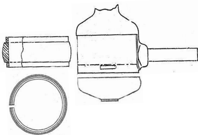
Bild 12.54: Zeichnungen im Patent P.A. 491797 vom 27.08.1958
