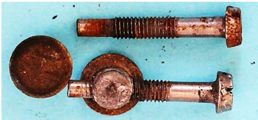
Bild 10.22: Elemente zur Verschraubung der Gehäuseteile
