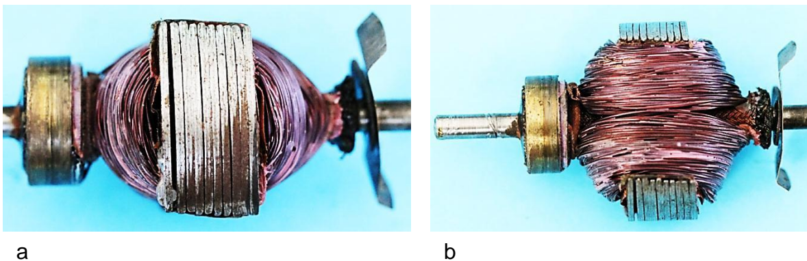
Bild 9.20: Doppel-T-Anker: a) Polfläche, b) Pollücke
