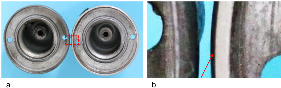
Bild 6.9: Nachweis der Aluminiumkappe an der Lagerhalskante: a) Lagerhalsfüße der Dynamos Impex 30 und Impex-Super, b) Roter Ausschnitt von a
