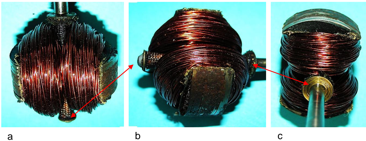
Bild 9.27: Bewickelter Doppel-T-Anker: a) Ansicht der Spulenseiten, b) Polfläche des Ankerblechpakets, c) Wicklungsköpfe und Masseschleifscheibe
