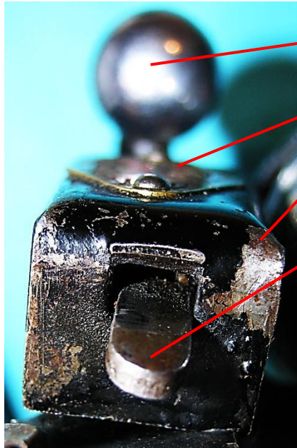
Bild 2.9: Führung des Stö- ßels im Schlitz des Basis- blechs
