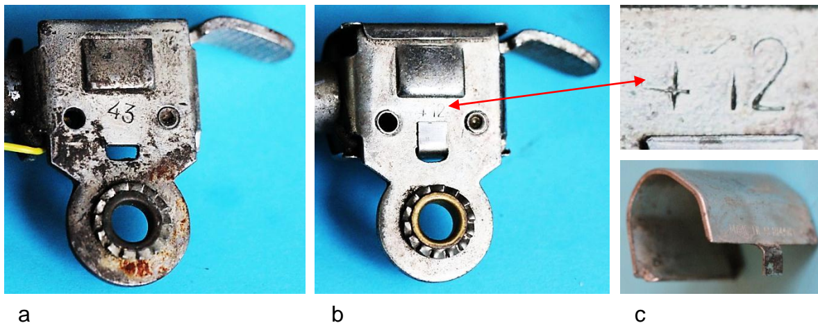
Bild 12.72: Nummerierung auf der Rückseite der Kippvorrichtung des K-10817 (400): a) Nummer 43, b) Nummer 412, c) Form des Abdeckblechs
