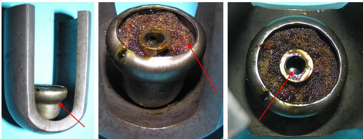
Bild 6.33: Drei Ansichten des Spurlagers: a) Lagertopf auf der Innenseite des Jochs, b) Öldepot, c) Kugel zur axialen Abstützung
