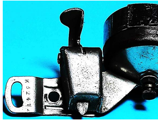
Bild 12.31: Kippschalterprinzip: a) Boden mit Kabelanschlussbolzen und angenietetem Flansch der Kippvorrichtung, b) Kippvorrichtung mit der K-Nummer K 32412
