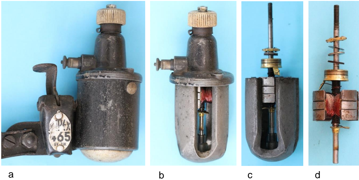
Bild 10.5: Baugruppenkombinationen: a) Gesamtansicht, b) Generator mit Lagerhals, c) Anker und vierpoliger Magnet, d) Anker mit dem Schleifring
