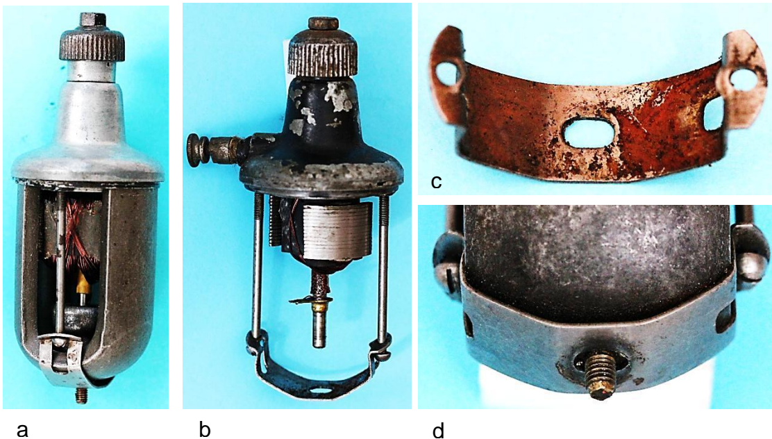
Bild 7.17: Spannelemente zur Befestigung des Magneten am Lagerhalsfuß
