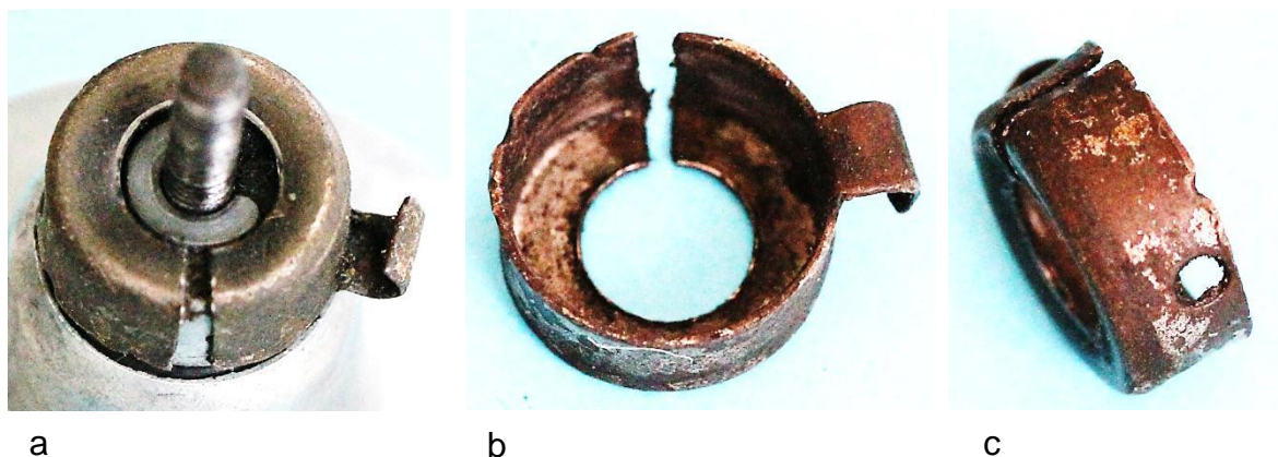
Bild 7.12: Verschlusskappe der Ölbohrung
