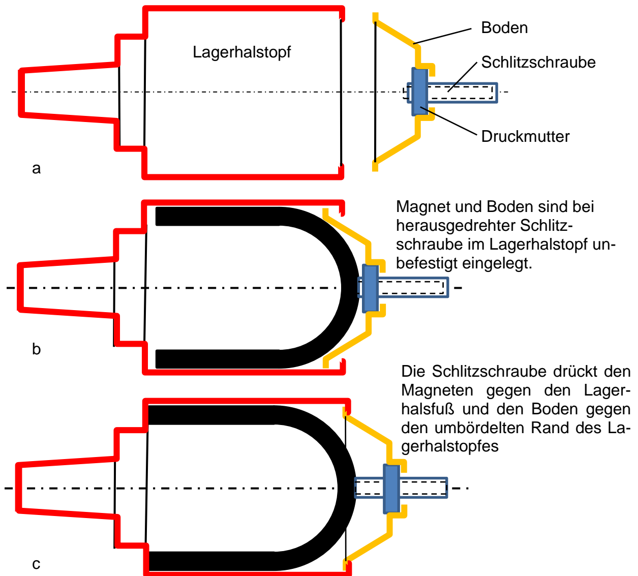
Bild 9.18: Vereinfachte Darstellung des Fügevorgangs der Gehäuseteile
