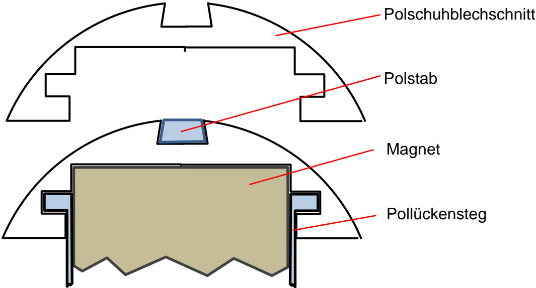
Bild 12.19: Querschnitt eines Polschuhs
