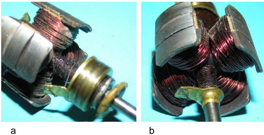
Bild 10.9: Vierpoliger Sternanker: a) Spannung führender Schleifring, b) Masseanschluss
