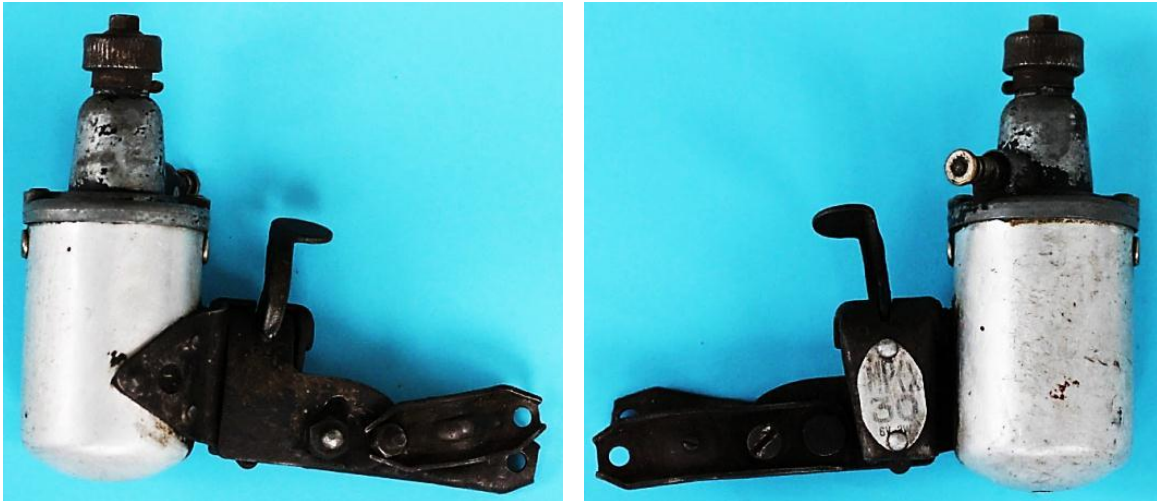
Bild 6.19: Impex 30: 6 V; 3 W, Fertigungsnummer K 34320
