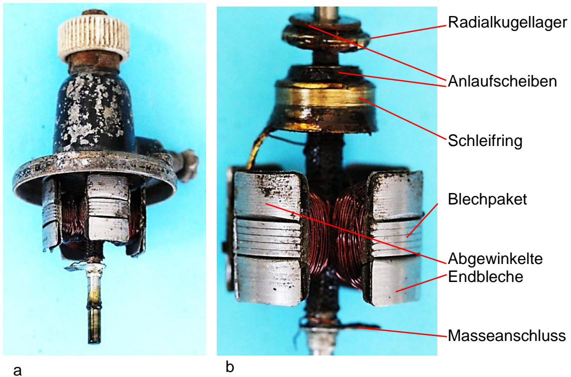
Bild 10.26: Anker: a) Anker im Lagerhals eingefügt, b) Bauteile des Ankers
