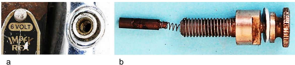
Bild 9.13: Spannung führender Kontakt: a) Gewindeeinsatz im Gehäusemantel, b) Kombination aus Bürstenhalter und Kabelanschlussbolzen mit Bürste
