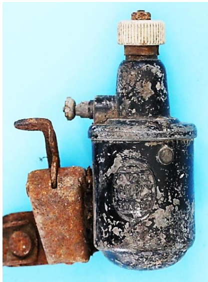
Bild 10.24: Vierpoliger Magnet: a) Dynamokörper, b) Am Lagerhalsfuß angespresster Magnet, c) Firmenlogo der Magnetfabrik Bonn
