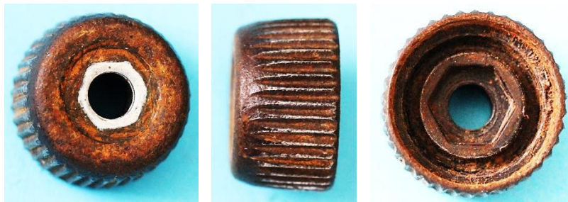
Bild 12.48: Reibräder: a) Stahlreibrad mit Innengewinde, b) Keramikreibrad c) Stahlkappe mit Innensechskant
