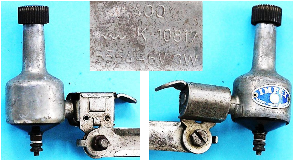
Bild 12.69: Impex K-10817 (400) Typ 5554
