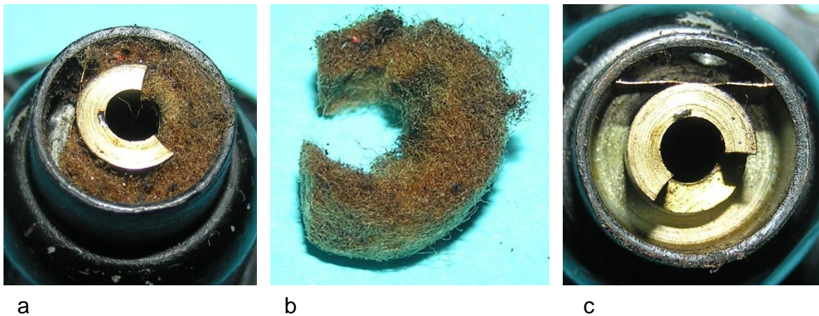
Bild 6.37: Öldepot im oberen Rand des Lagerhalses
