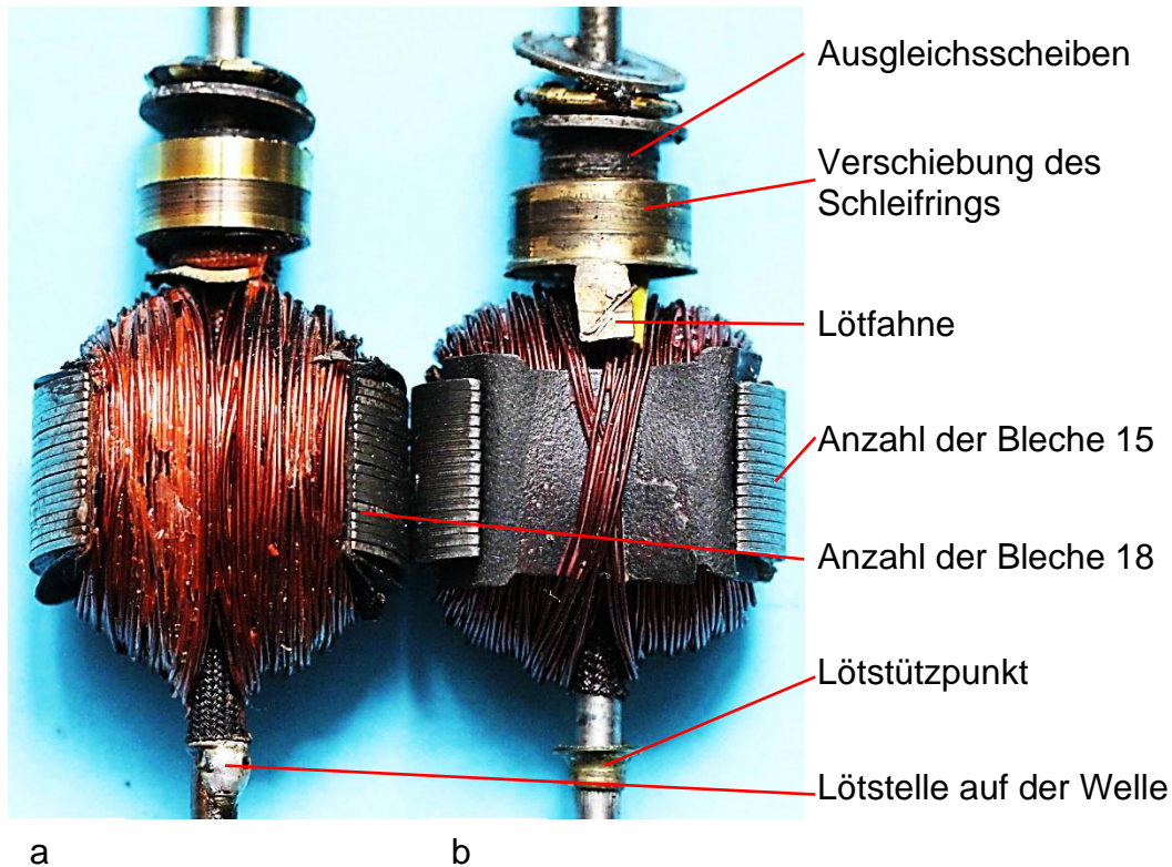
Bild 6.11: Konstruktive Unterschiede der Anker: a) Impex-Saba, b) Impex-Super
