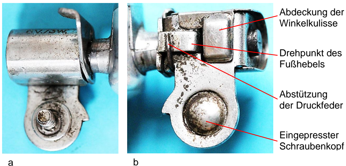
Bild 12.62: Kippvorrichtung: a) Abdeckblech, b) Rückseite
