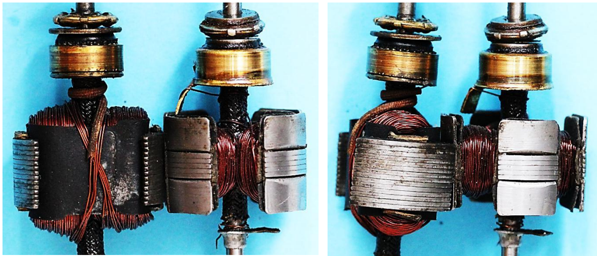
Bild 10.31: Vergleich zwei- und vierpoliger Anker: a) Pollücken, b) Polflächen
