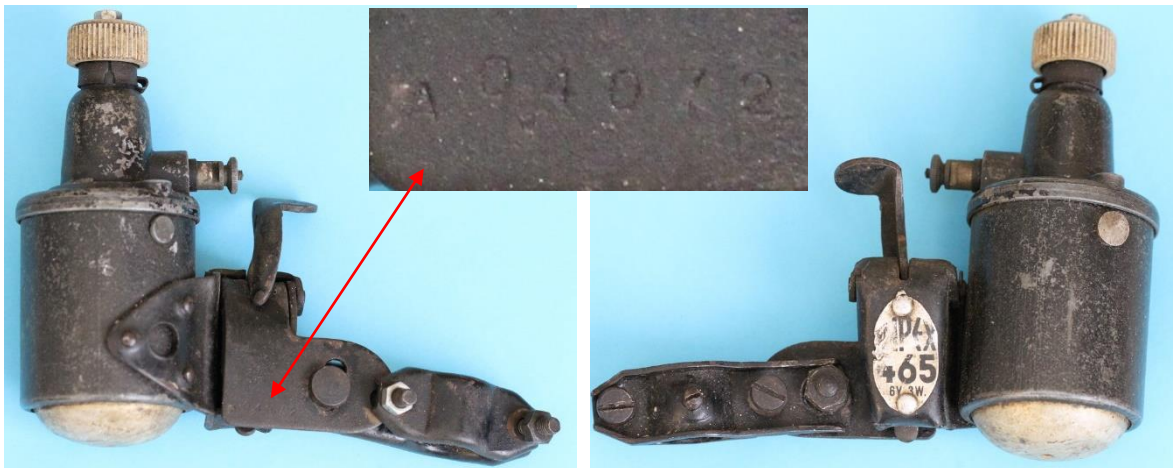
Bild 10.1: 3 W- Impex-Dynamo Typ 465 mit dreiteiligem Gehäuse und der Fertigungsnummer A 04072
