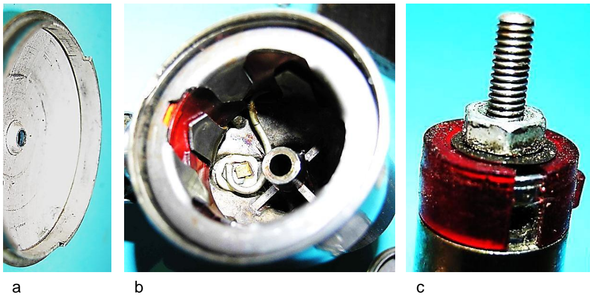
Bild 12.37: Baugruppen: a) Boden, b) Anker, c) Öllochabdeckung
