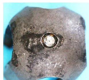
Bild 10.25: Spurlager: a) Ansicht durch eine Pollücke, b) Magnetjoch mit angenietetem Spurlager
