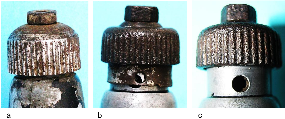
Bild 7.11: Unterschiede bei der Abdeckung des Öllochs: a) Padena, b) Impex 21 mit Öllochverschlusskappe, c) Impex 21 ohne Öllochverschlusskappe
