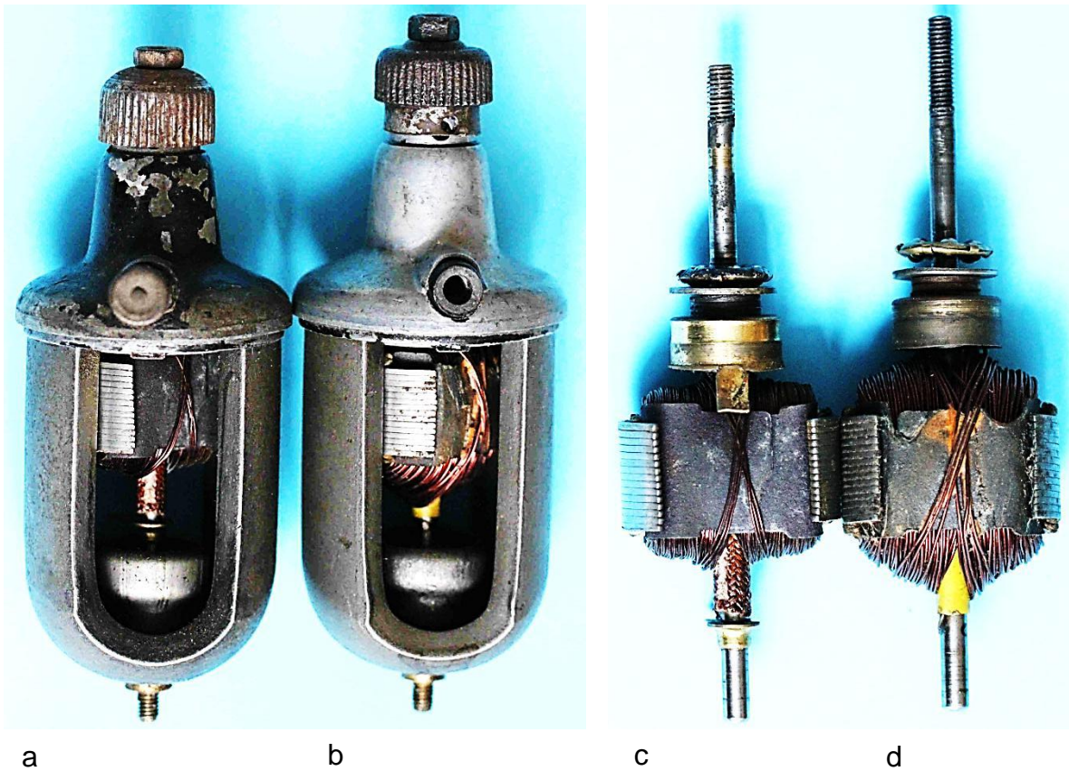
Bild 7.18: Vergleich des Impex 21 mit Padena: Entfernter Gehäusetopf: a) Padena, b) Impex 21; Ankervergleich: c) Padena, d) Impex 21
