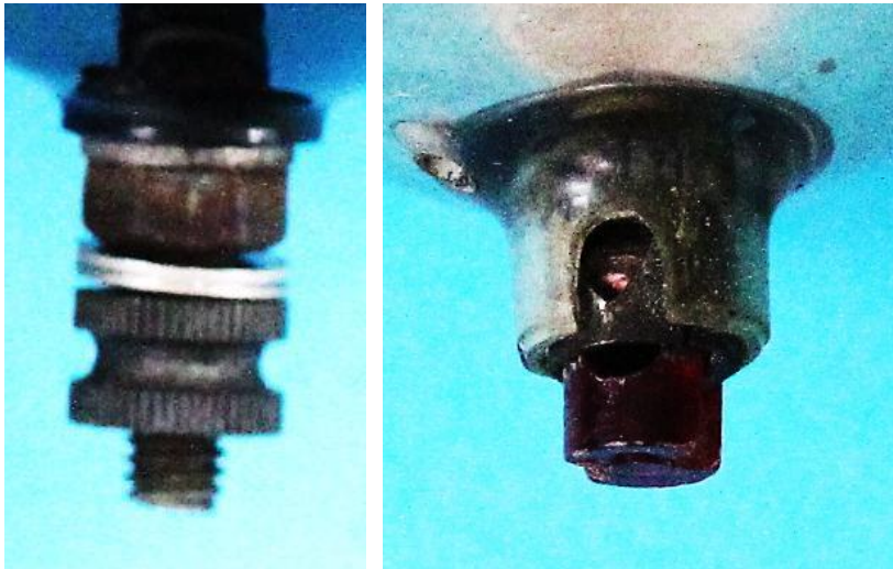
Bild 12.76: Kabelanschlüsse durch Schraub- und Federklemmen
