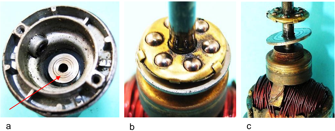
Bild 7.15: Axiallager: a) Obere Anlaufscheibe im Lagerhals, b) Axialkugellager, c) Untere Lagerscheibe
