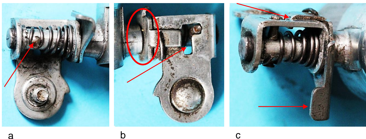
Bild 12.63: Kippvorrichtung in der Ruhestellung: a) Abstützung der Druckfeder am Sperrstift, b) Winkelkulissee mit Sperrstift, c) Drehpunkt und Krafrichtung beim Entriegeln
