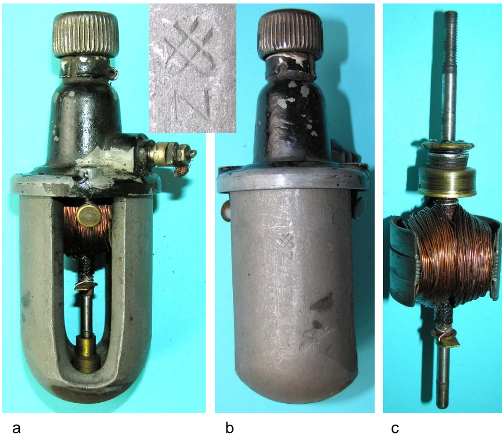
Bild 6.24: Generator: a) Blick durch die Pollücke zum Anker, b) Gestempelter Magnetschenkel, c) Läufer
