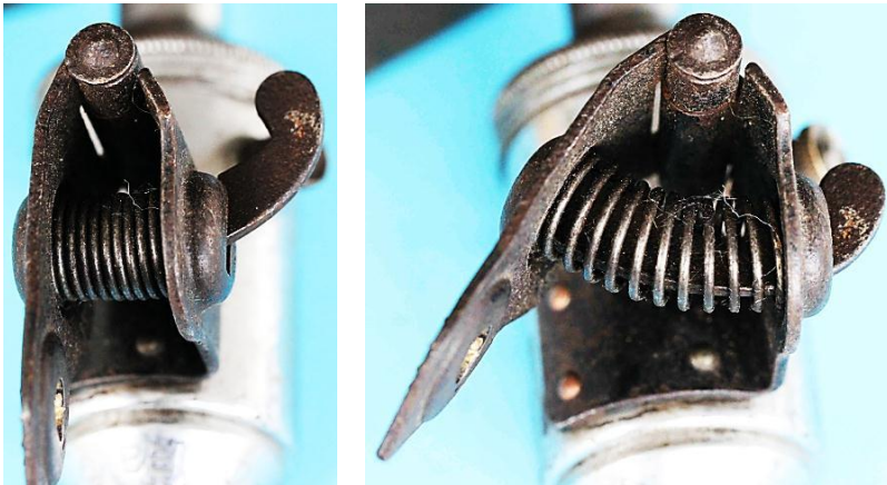
Bild 2.1: Berko-Kippvorrichtung
