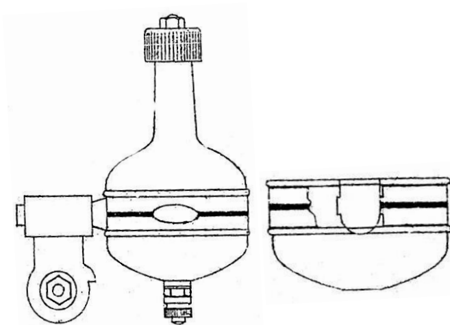
Bild 12.53: Zeichnungen im Patent P.A. 03258C vom 17.01.1956
