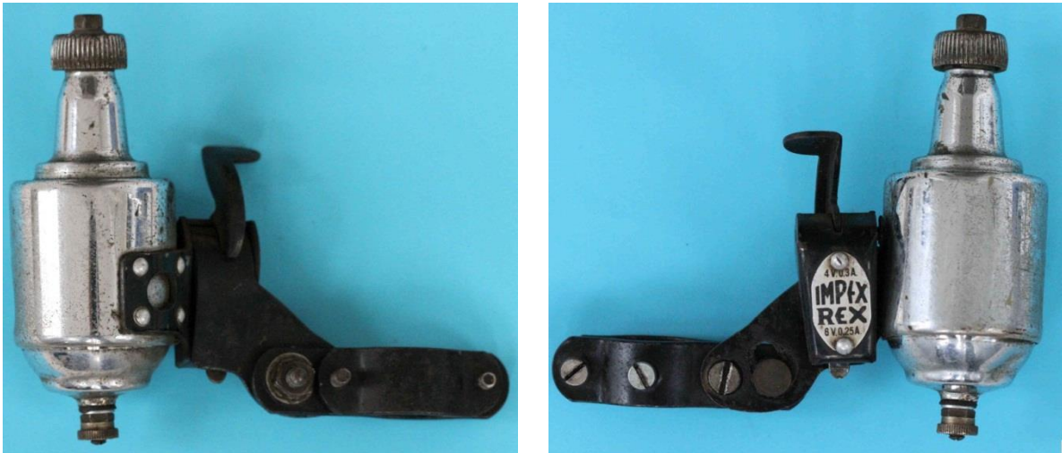
Bild 9.24: Impex-Rex mit dem Kabelanschlussbolzen im Boden
