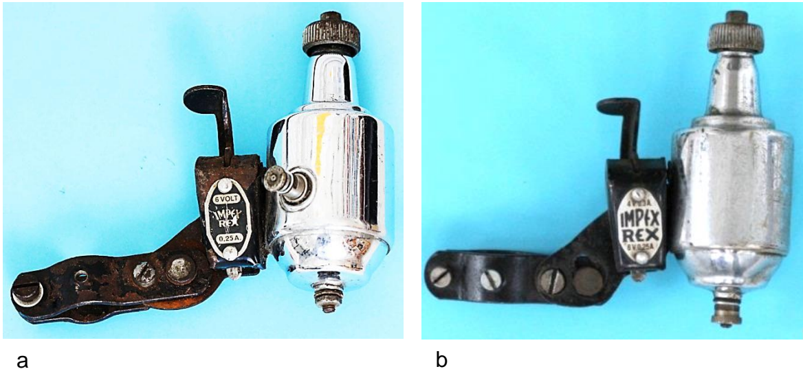
Bild 3.7: Impex Rex: Zweipoliger Tulpenmagnet-Dynamo mit umbördeltem Lagerhalstopf für 1,5 W: a) Kabelanschluss am Gehäusemantel, Nr. E 02440, b) Kabelanschluss am Boden, Nr. E 34627, Gewicht je 460 g.
