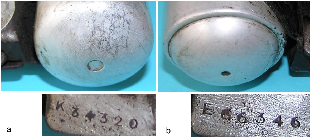
Bild 6.23: Unterschiede in der Bodenform: a) Impex 30, K 34320, b) Impex 30, E 66346
