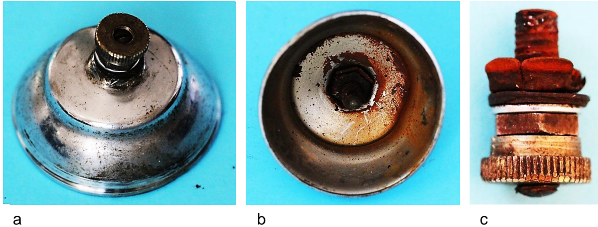
Bild 9.26: Boden: a) Kabelanschlussbolzen im Boden, b) Verdrehsicherer Sitz der Druckmutter, c) Spanschraube bzw. Kabelanschlussbolzen
