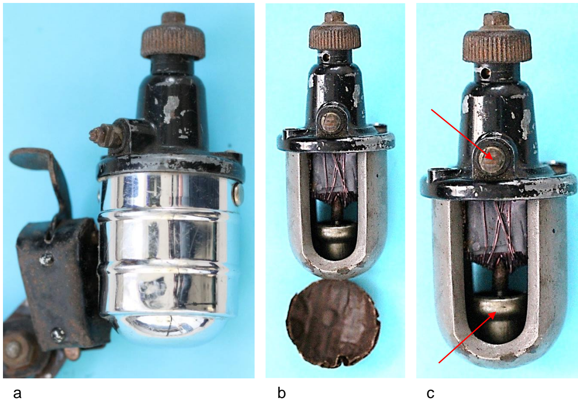
Bild 6.30: Ausrüstung mit einem zweipoligen Tulpenmagneten: a) Nach unten gewölbter Boden, b) Anpassung des Magnetjochs an die Bodenkrümmung mit einer Papierzwischenlage, c) Kabelanschlussbolzen und Spurlager
