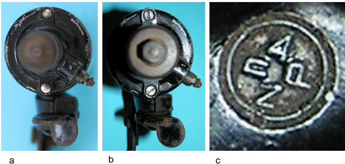
Bild 6.28: Lagerhalsfußgestaltung: a) Abdeckung der Schraubenköpfe mit Messingkappen, b) Eingegossener Stempel mit den Initialen APZU oder VPZU oder 4PZU
