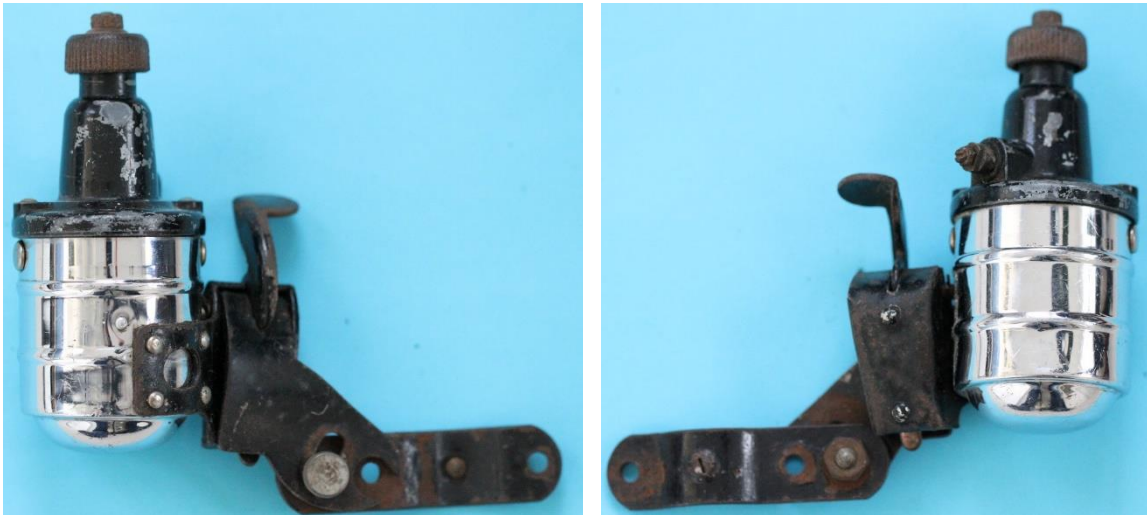
Bild 6.27: Zweipoliger Dynamo mit zwei nach außen gewölbten Ringnuten im Gehäusemantel, Fertigungsnummer B 24836
