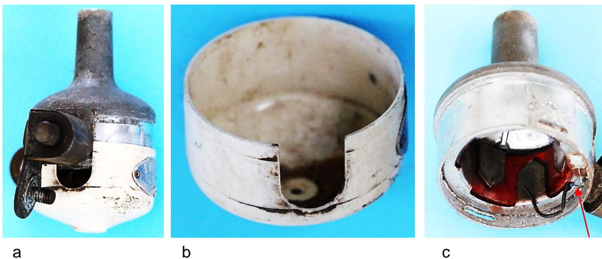
Bild 12.56: Zweiteiliges Gehäuse: a) Ineinander geschobene Gehäuseteile, b) Gehäusetopf aus Duroplast, c) Klauenpole des Ankers mit Lötstelle für den Masseanschluss
