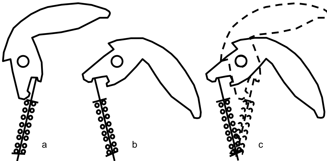
Bild 7.23: Endstellungen der Kippeinrichtung: a) Ruhestellung, b) Betriebsstellung, c) Vergleich beider Stellungen
