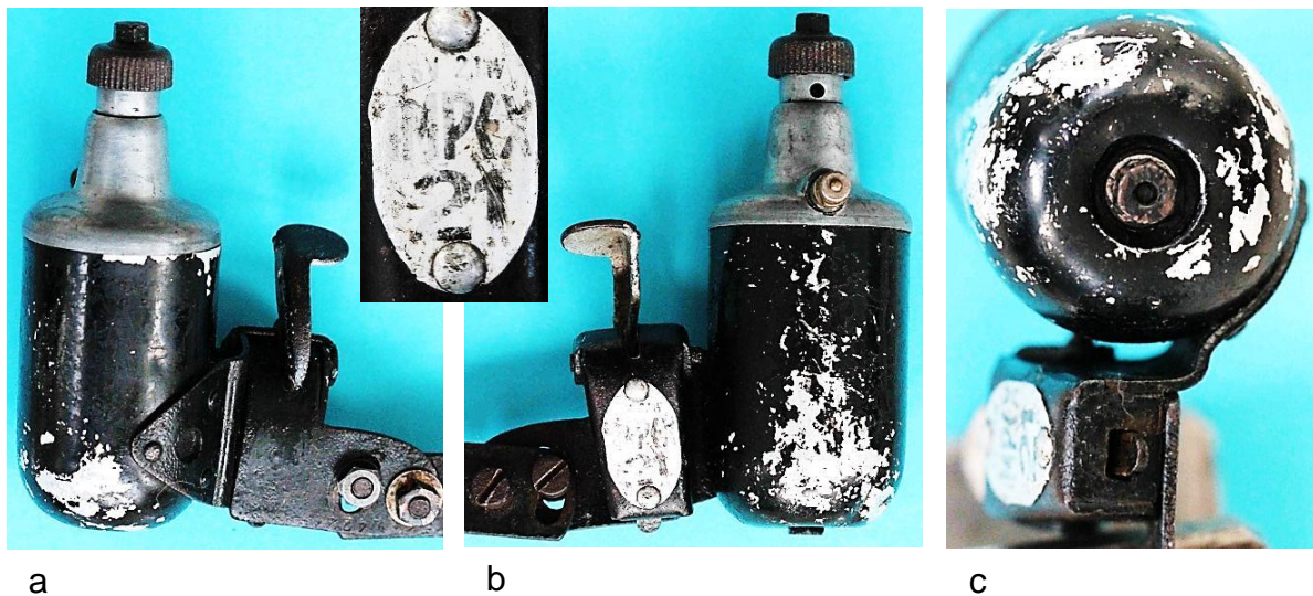
Bild 7.6: Impex 21: a) Rückseite, b) Vorderseite, c) Boden
