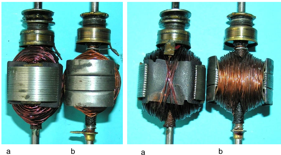
Bild 6.26: Gegenüberstellung der beiden Läufer: a) Impex 30, K 64320, Gewicht 100 g, b) Impex 30, E 66346, Gewicht 57 g
