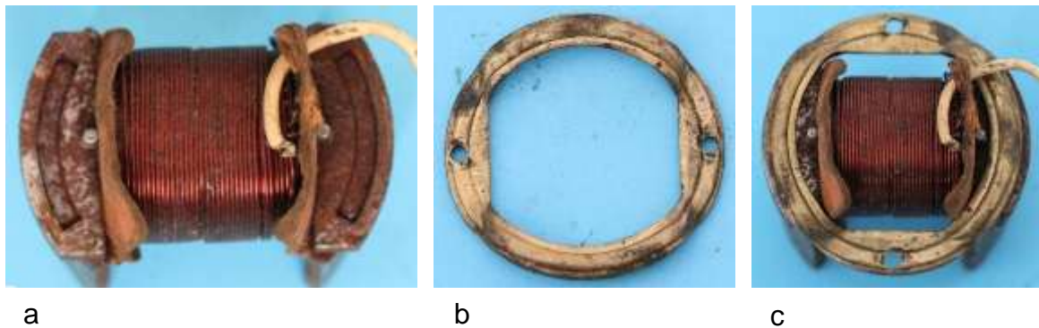
Bild 2.8: Ring zur Befestigung des Ankers: a) Unterseite des Ankers, b) Spannring, c) Position des Spannringes auf dem Anker
