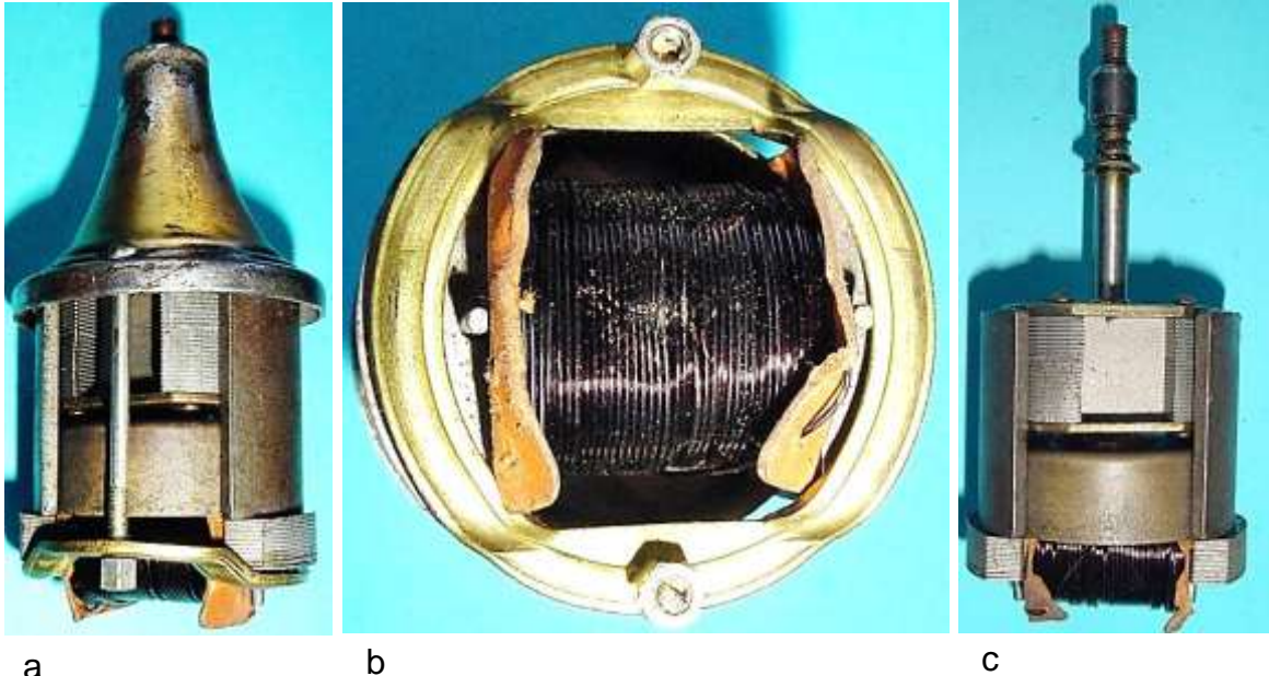
Bild 2.7: Aufbau des Generators: a) Lagerhals mit Generator, b) Ankerspule, c) Anker und Polrad
