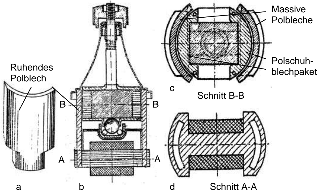
Bild 2.3: Zeichnungen im französischen Patent Nr.782.180 von M. Albert, Joseph, Gaston .Huyghe: a) Polblech, b) Gesamter Querschnitt, c) Querschnitt durch das Polsystem; Anmeldedatum: 28.11.1934
