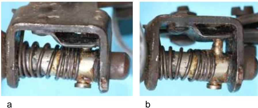
Bild 1.4: Kippvorrichtung von oben: a) Arbeitsstellung, b) Ruhestellung
