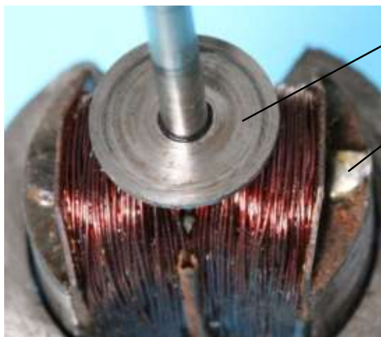
Bild 1.10: Massekontakt: a) Anker mit Welle und Reibrad, b) Auf der Welle leitend befestigtes Schleifrad
