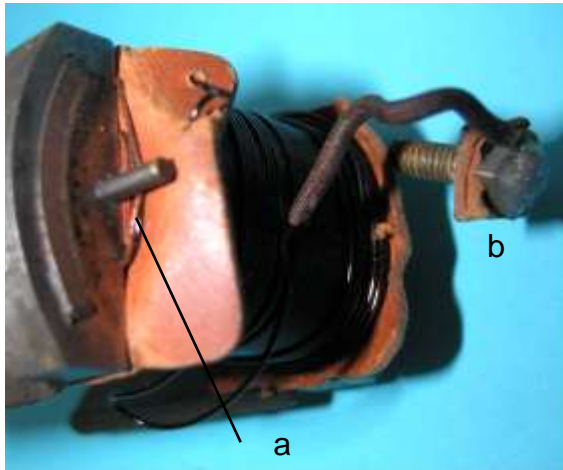
Bild 3.12: Spulenanschlüsse: a-Massekontakt b-Anschluss am Kabelbolzen
