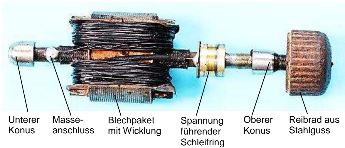
Bild 2.7: Vollständiger Rotor
