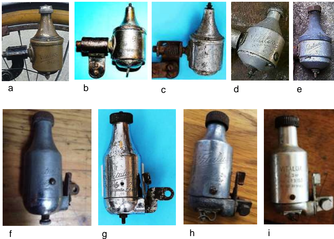
Bild 1.2: Übersicht der Vitaluxdynamos, die nach den zweipoligen Tulpenmagnetdynamos auf den Markt kamen: Die Muster b), c) und g) stehen für eine Analyse zur Verfügung, die übrigen Ausführungen entsprechen Darstellungen im Internet
