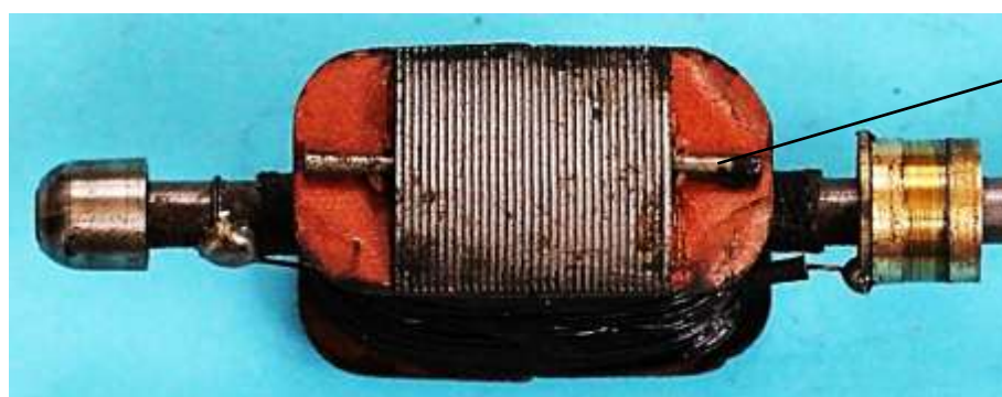
Bild 2.9: Spulenanschlüssen, Schleifkontakte und Wicklungskopfstab
