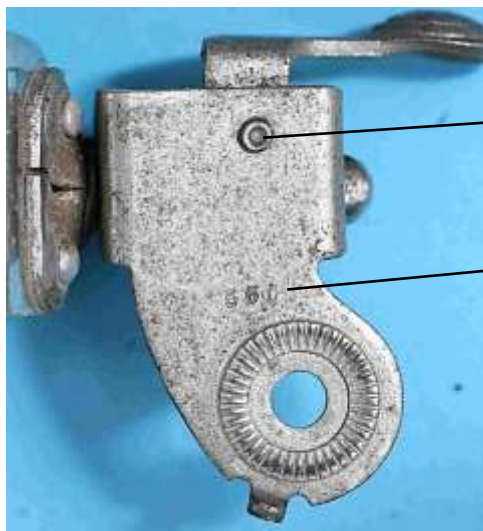
Bild 2.3: Rückseite der Kippvorrichtung mit eingprägter Nummer 560 und dem Drehpunkt des Fußhebels
