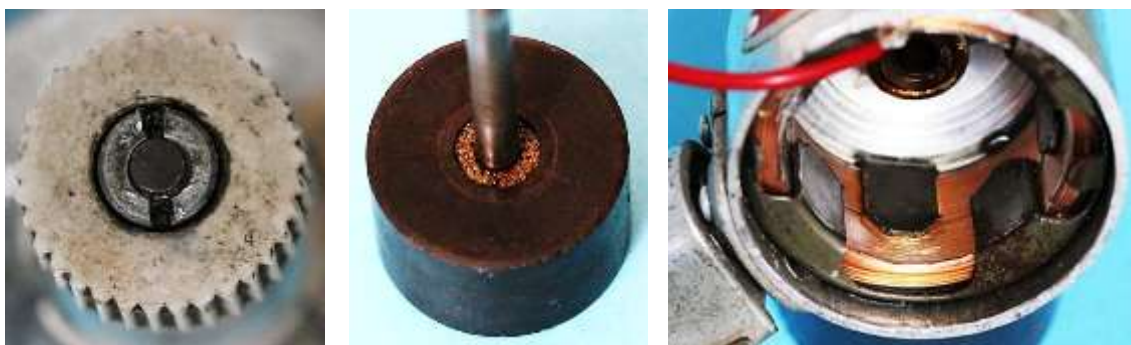
Bild 2.8: Generator: a) Reibrad mit versenkter Schlitzmutter, b) Polrad (30 mm Durchmesser, 18 mm axiale Länge), c) Klauenpolanker
