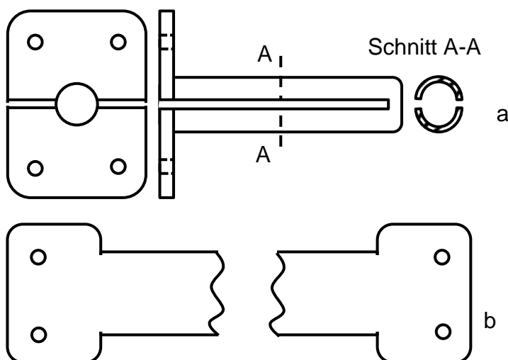
Bild 2.12: Skizzen zur Konstruktion des Drehbolzens a) Ansichten des Drehbolzens b) Ausgeschnittenes Blech
