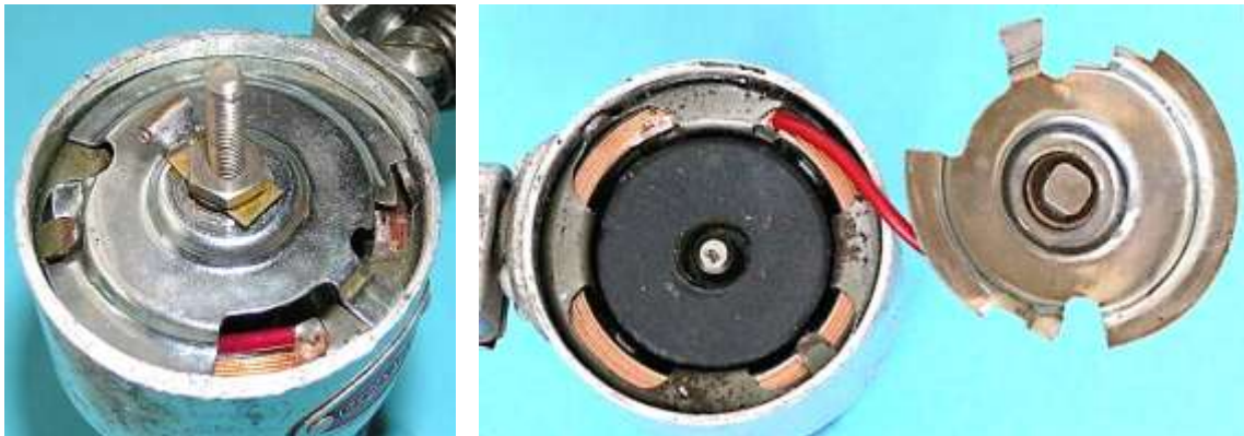
Bild 2.7: Aufgeklappte Kontaktplatte: a) Eingebaute Kontaktplatte, b) Stirnseite des Generators, c) Oberseite der Kontaktplatte
