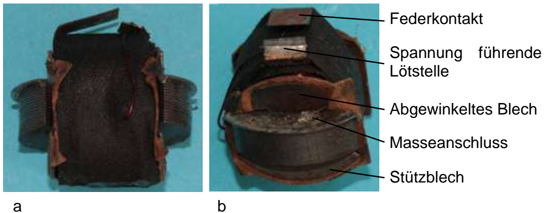
Bild 3.23: Ankerspule und geblechter Spulenkern
