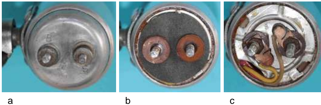
Bild 5.81: Kabelanschlussbolzen: a) Boden mit den Anschlussbezeichnungen B und S, b) Isolierung der Kontaktplatte, c) Kontaktplatte mit den Spulenanschlüssen
