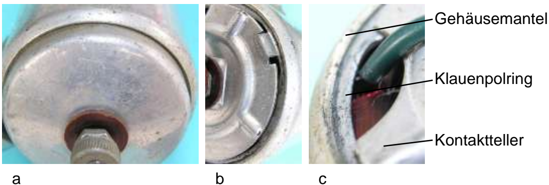
Bild 5.55: Bodenbefestigung: a) Angeschraubter Aluminiumboden, b) Eingehakter Kontaktteller, c) Klauenpoltring als Anlage für den Boden genutzt
