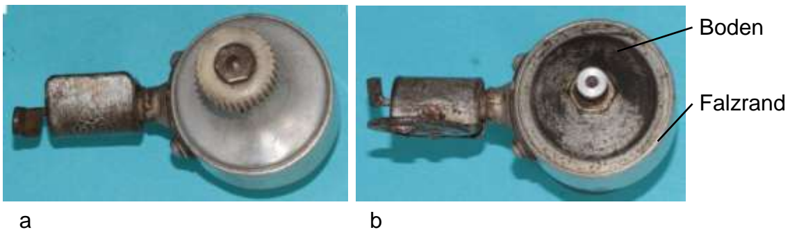
Bild 4.42: Ansichten: a) Lagerhals mit Reibrad, b) Eingefalzter Boden
