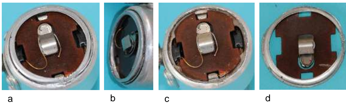
Bild 5.57: Kontaktplatte: a) und b) Mit dem Zwischenring befestigte Kontaktplatte, c) Zwischenring entfernt, d) Kontaktplatte mit Zwischenring
