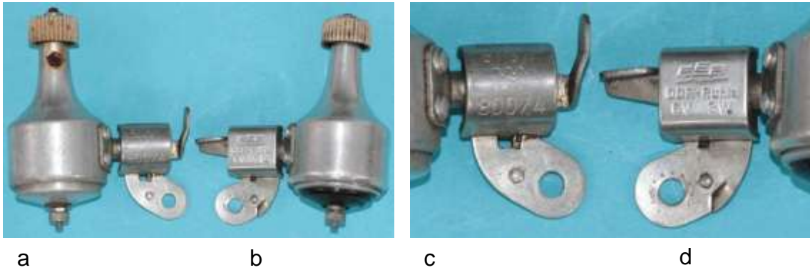
Bild 5.53: Sichtbare Veränderungen mindestens seit 1977 innerhalb der Serie 8007.4: Ölbohrung, Boden, Abdeckung der Kippvorrichtung, Bedienungshebel: a) Etwa bis 1977, b) Etwa ab 1977
