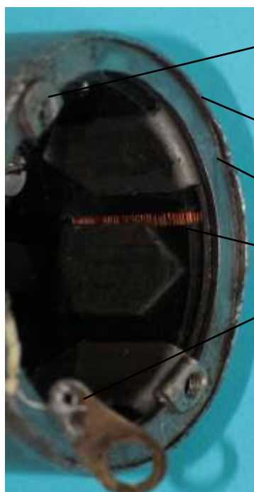
Bild 5.28: Ankerbauteile
