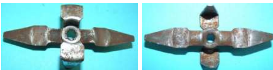
Bild 4.62: Zwei aufgebogenen Polschuhe eines Klauenpolrings
