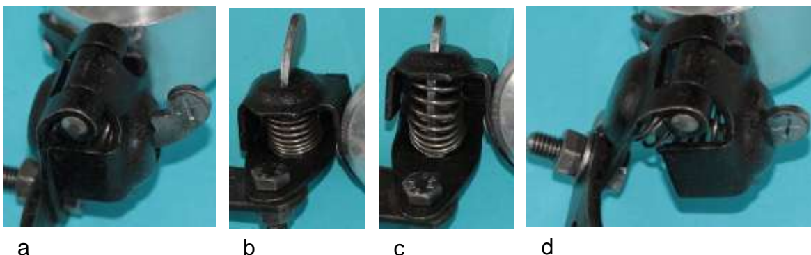
Bild 5.22: Kippvorrichtung: a) und b) Ruhestellung, c) und d) Betriebsstellung
