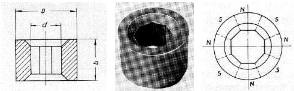
Bild 5.30: Walzenmagnet für Fahrraddynamos im Prospekt des VEB Keramische Werke Hermsdorf von 1956
