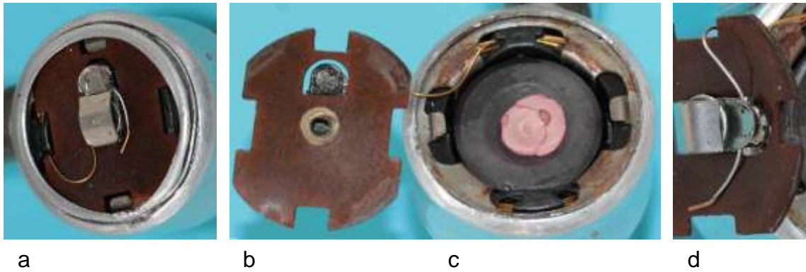
Bild 5.59: Kontaktierung: a) Mit einem Hohlkorn befestigte Blattfeder, b) Oberseite der Kontaktplatte, c) Zur Blattfeder geführtes Spulenanfang, d) In der Feder eingeklemmter Aluminiumdraht
