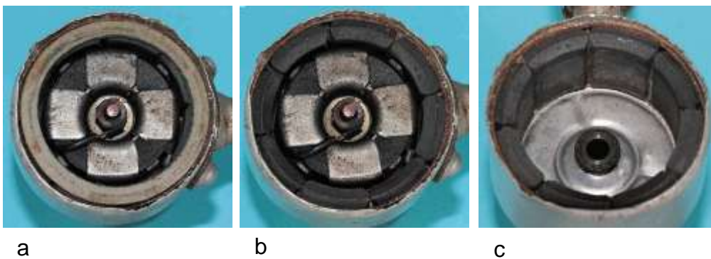
Bild 4.43: Magnetsystem: a) Abdeckung der Magnete mit einem Dichtungsring, b) Stirnseiten der Magnete mit Anker, c) Magnete und unteres Lagerschild
