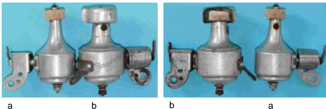
Bild 5.47: Gestaltungsänderung bei der Einführung der Serie 8007.4: a) Typ 8007.4, b) Standard 8007.3
