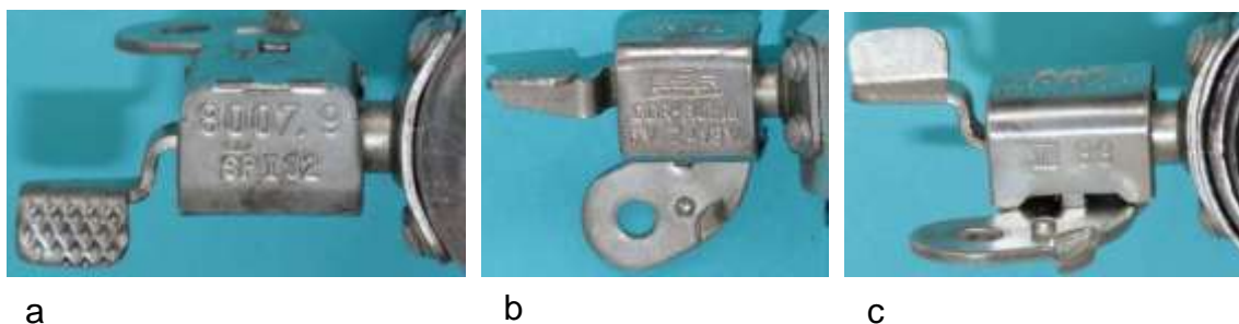
Bild 5.84: Abkröpfung des Fußpedals: a) Ansicht von oben, b) Seitenansicht, c) Ansicht von unten
