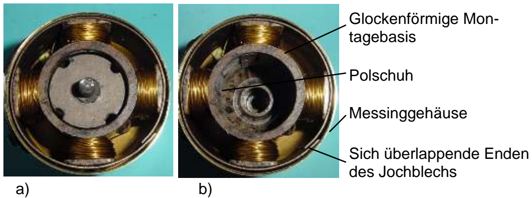
Bild 3.59: Elektromagnetischer Kreis: a) Läufer mit Anker, b) Innenansicht der Duroplastkonstruktion
