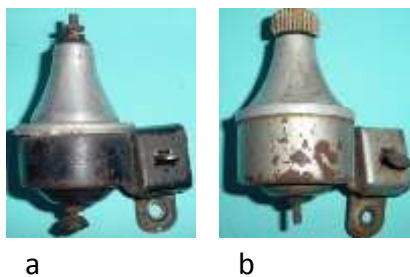
Bild 1.3: Balaco-Dynamos mit acht Keramikmagnetblöcken und rotierendem Klauenpolanker a) 2,1 W b) 3 W,
