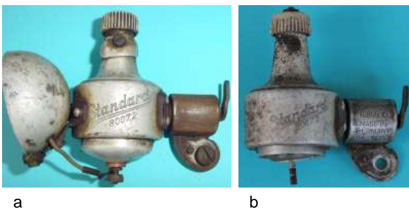
Bild 4.56: Vergleich: a) Standard 8007.2 b) Standard 8007.3
