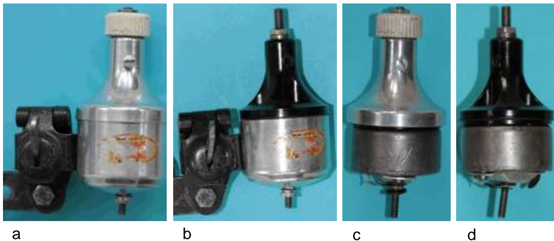
Bild 5.23: Gehäuse: a) Gehäuse bestehend aus Gehäusetopf und Lagerhals, b) Äußerer Lagerhals entfernt, c) Gehäusetopf entfernt, d) Dynamo ohne Gehäuse
