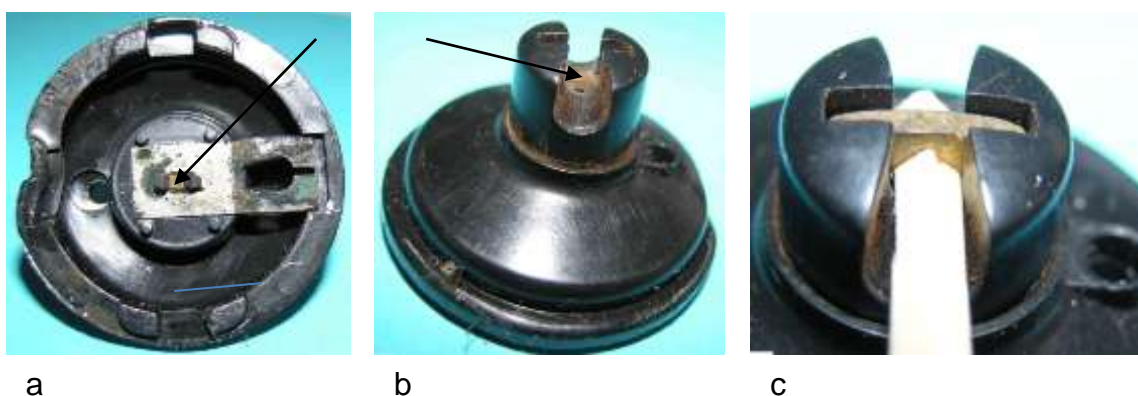
Bild 5.71: Kabelanschluss: a) Boden mit Schneidklemme, b) Druckknopf, c) Eingeklemmtes Anschlusskabel
