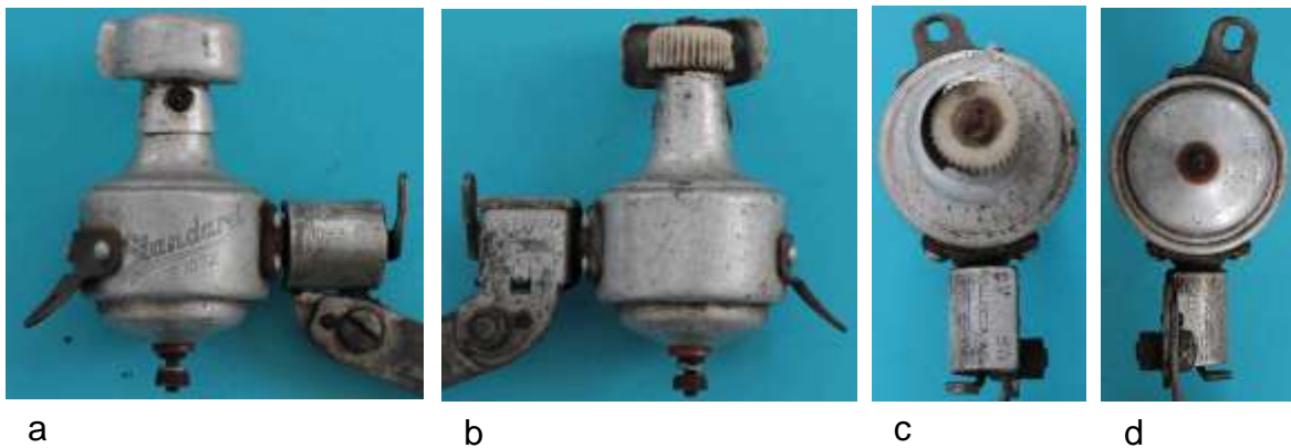
Bild 4.46: FER Standard 8007.2
