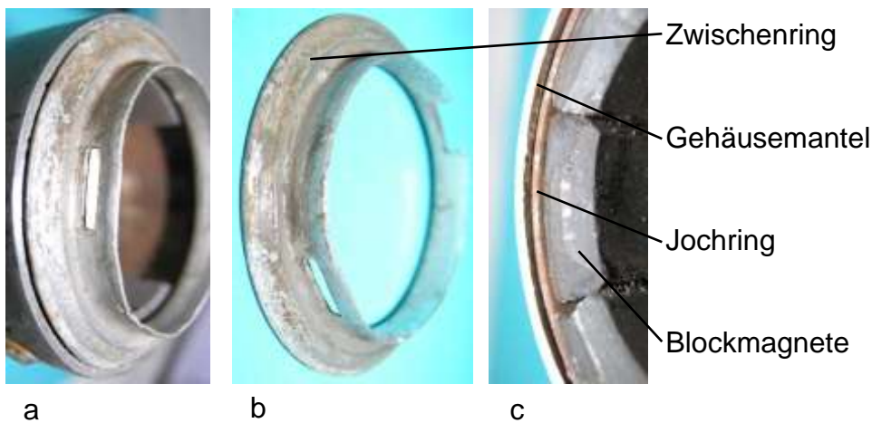
Bild 4.55: Zwischenring: a) Position des Zwischenrings nach Entfernung der Umbörtelung des Gehäuses, b) Zwischenring, c) Stirnseite des Jochrings, die Auflagefläche des Zwischenrings
