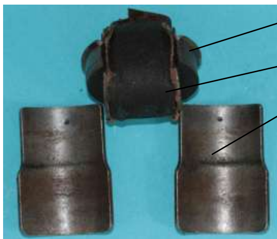
Bild 3.22: Anker, Spule, Blechpaket und Pol-schuhe
