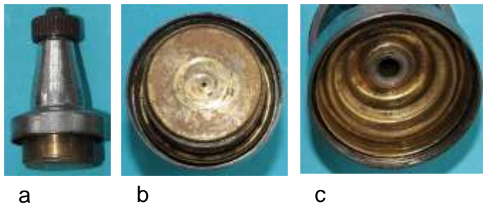
Bild 3.27: Lagerhals a) Lagerhals mit Polrad, b) Untere Ansicht des Polrades c) Lagerteller mit Lagerrohr
