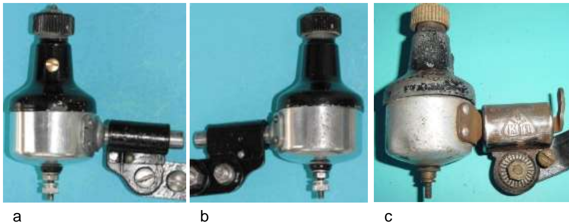
Bild 3.28: Melas 6 V; 2,1W im Vergleich mit der Ausführung IKA-FEK
