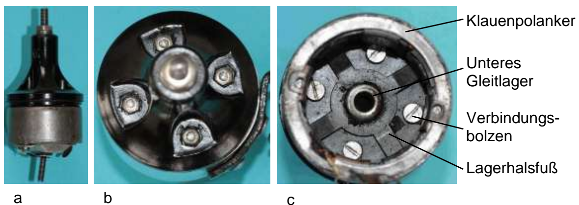
Bild 5.24: Verschraubung des inneren Lagerhalses mit dem Ankerjoch: a) Seitenansicht der Generatorbaugruppe, b) Vier Muttern in Vertiefungen auf der Reibradseite, c) Schraubenköpfe auf der Ankerseite
