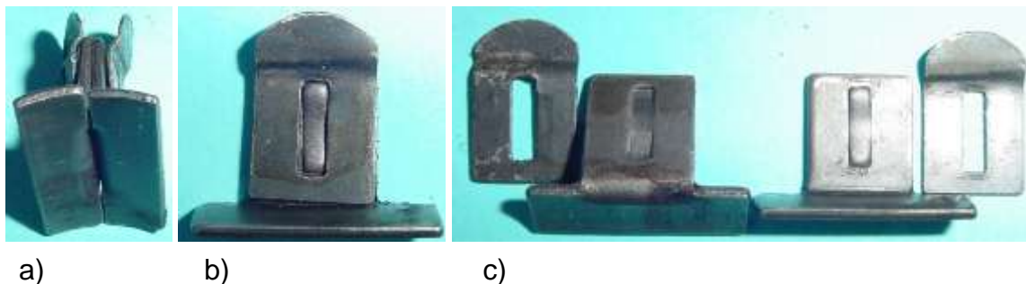
Bild 3.60: Pol mit Spulenkern: a) Gesamtansicht, b) Ineinander gefügtes Blechpaar, c) Einzelteile des Pols
