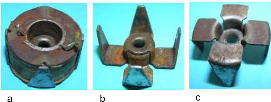
Bild 4.61: Anker: a) Spule mit ferromagnetischem Kern, b) und c) Zusammengesetzte Klauenpolringe
