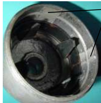
Bild 5.38: Anker, a) Ankerspule mit einem Klauenpolring, b) Bearbeitete Schiebeflächen
