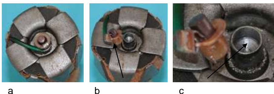
Bild 4.37: Spannung führender Schleifkontakt: a) Spulenanschluss, b) Isoliert eingesetzte Kupferbürste, c) Grundbohrung in der Welle
