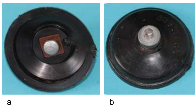
Bild 5.58: Boden: a) Innenseite b) Kabelanschlusseite
