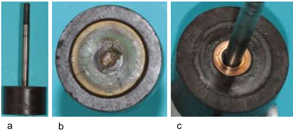
Bild 5.29: Polrad: a) Walzenmagnet mit Welle, b) Magnet mit Kunststofffüllung , c) Obere Polradseite mit Anlaufscheibe
