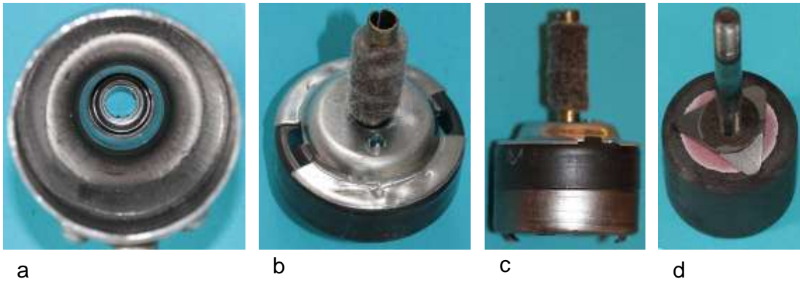
Bild 5.93: Montageeinheit aus Anker und Lager: a) Innenansicht des Lagerhalstopfs, b) Am Klauenpolring eingeklinktes Lagerschild, c) Vollständige Montageeinheit aus Anker und Lager, d) Achtpoliges Polrad
