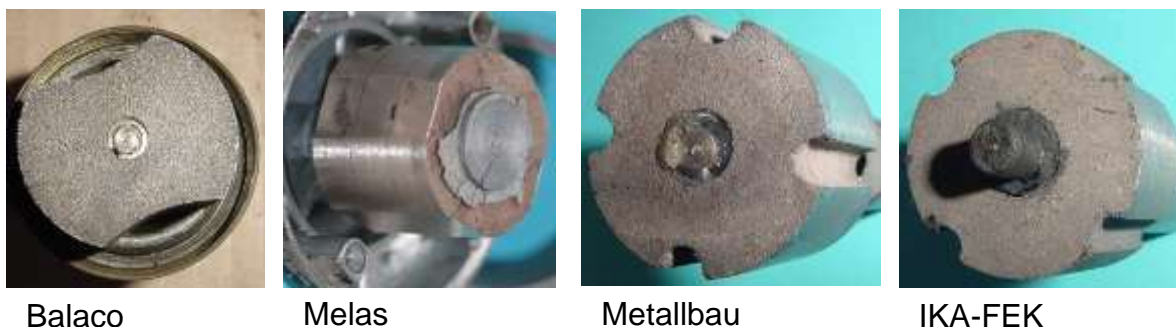
Bild 3.2: Ausgeführte AlNi-Polräder
