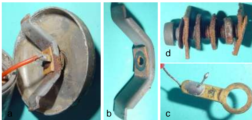
Bild 5.35: Kabelanschluss: a) Montagebügel mit Kabelbolzen und Boden, b) Montagebügel, c) Geschlossener Kabelschuh, d) Kabelbolzen mit Isolierscheiben
