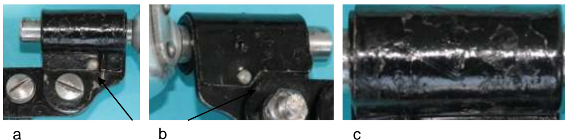
Bild 3.29: Kippvorrichtung: a) und b) Angenietetes Abdeckblech, c) Beschriftung auf dem Abdeckblech, 6 V, 2,1 A, Firmenlogo mit der Markenbezeichnung Melas
