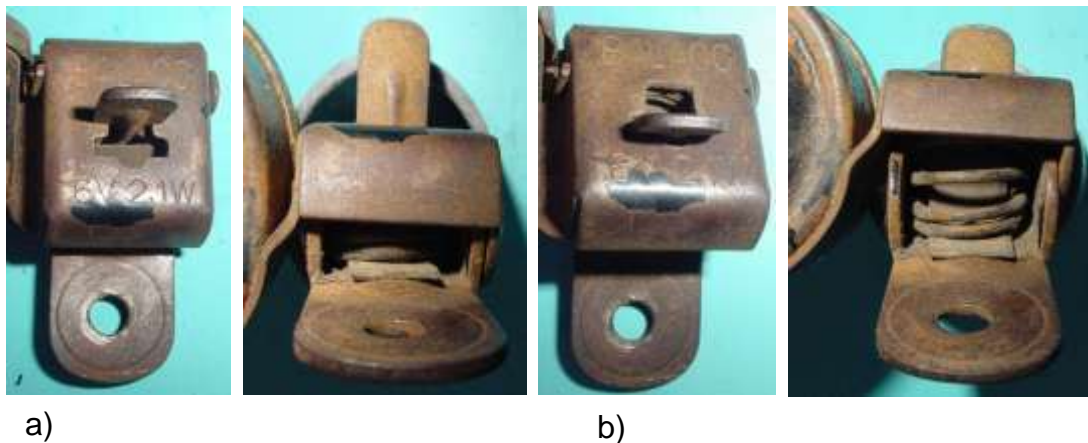
Bild 4.10: Kippvorrichtung: a) Arretierte Stellung, b) Andruckstellung
