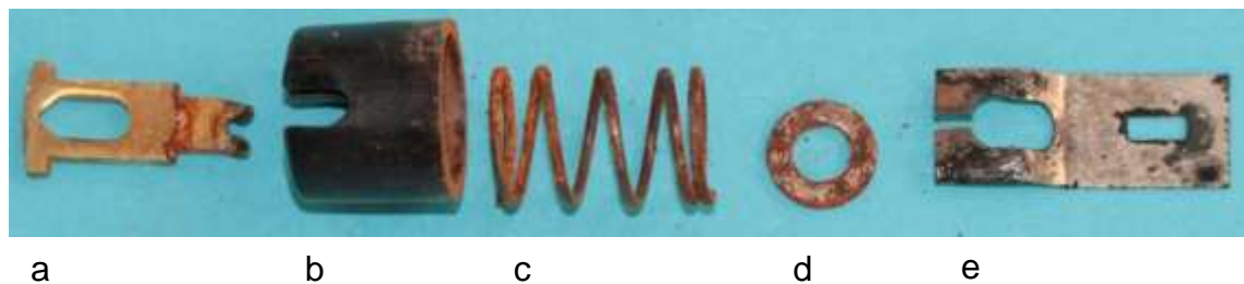
Bild 5.73: Kabelanschlusskontakt: a) Kabelanschlussblech, b) Druckknopf, c) Druckknopffeder, d) Spreizscheibe, e) Schneidkontakt
