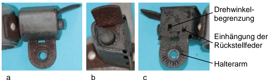
Bild 5.32: Kippvorrichtung: a) Abdeckung, Flansch und Bedienungshebel, b) Drehbolzen und Bedienungshebel, c) Basisblech mit Halterarm
