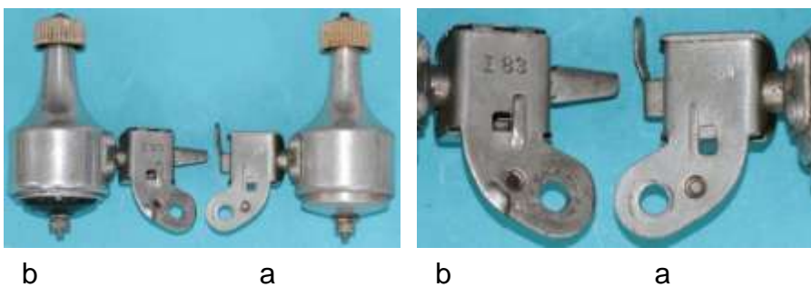
Bild 5.62: Fertigungsdaten auf dem Basisblech: a) 1964, b) 1983
