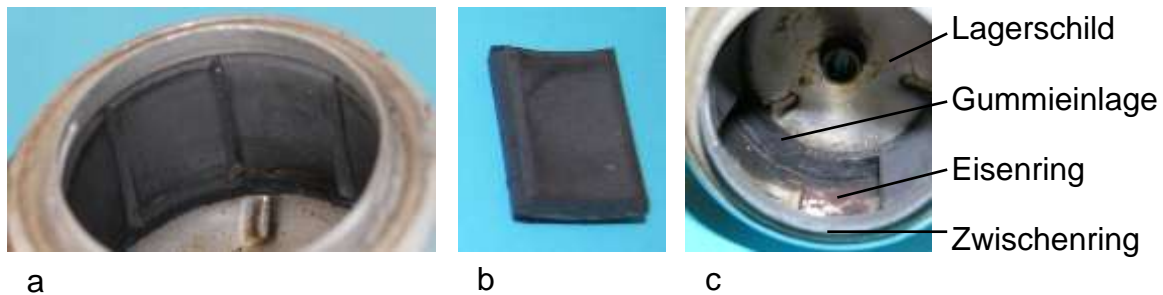
Bild 4.38: Magnetpolssystem: a) Acht Blockmagnete an der Gehäusewand positioniert, b) Blockmagnet 20 \times 15 \times 5 \text{ mm}^3 , c) Zwei Blockmagnete entfernt
