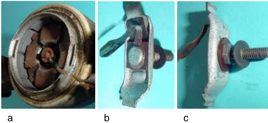
Bild 4.54: Spannung führender Kontakt
