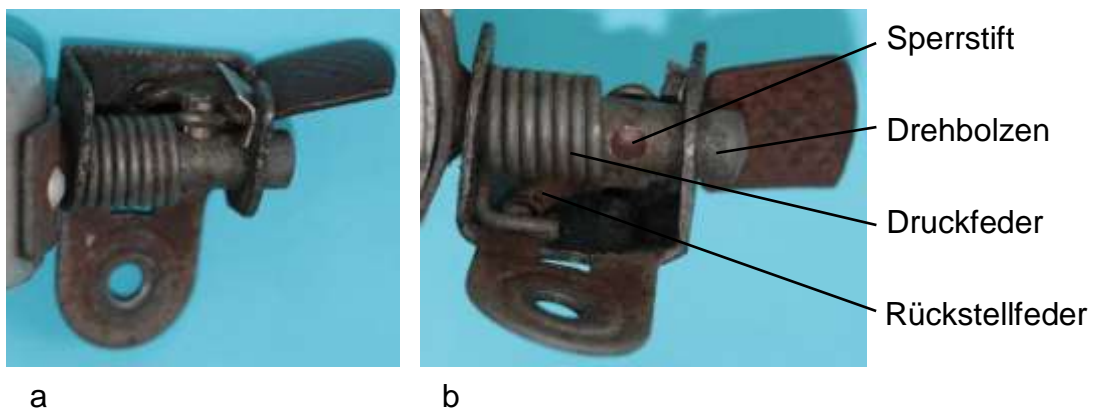
Bild 5.34: Ansichten in den zwei Stellungen: a) Ruhestellung, b) Betriebsstellung
