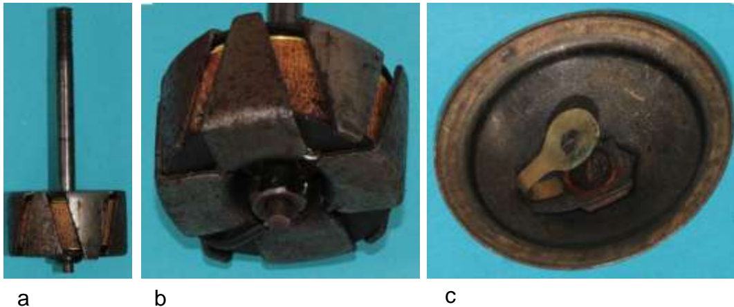
Bild 4.44: Anker: a) Klauenpolanker mit Welle, b) Bürste in der Stirnseite der Welle, c) Spannung führender Federkontakt
