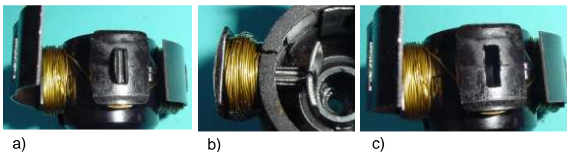
Bild 3.61: Position des Poleisens im Duroplastkörper: a) Aufgeklapptes Joch, b) In die Ständerbohrung verschobener Polschuh, c) Öffnung im Duroplastkörper für den Einsatz des Polschaftees
