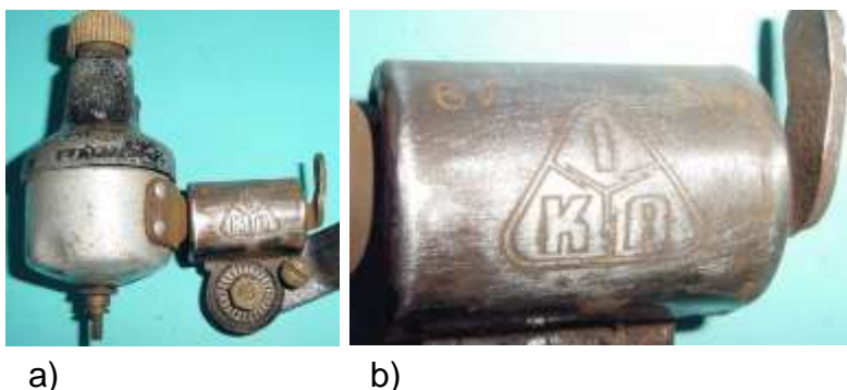
Bild 2.1: Dynamo mit kunststoffgebundenen Blockmagneten im Ständer
