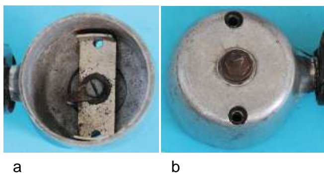
Bild 3.43: Bodentopf: a) Kabelanschluss innerhalb des Bodentopfes, b) Kabelanschluss außerhalb des Gehäuses
