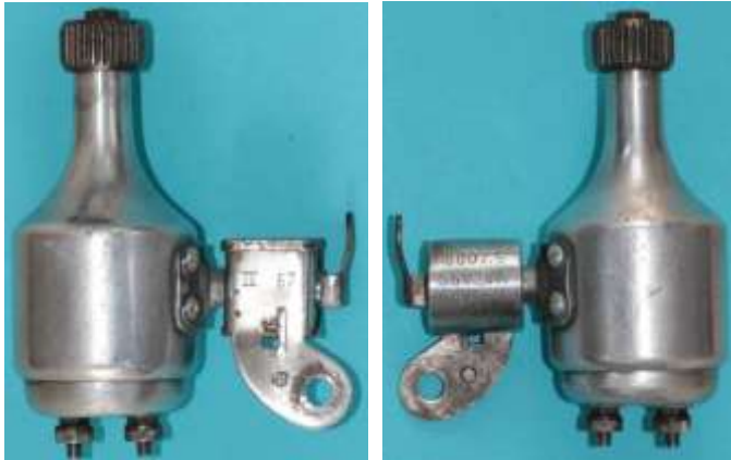
Bild 5.78: Parallelsystem 8007.5/1967
