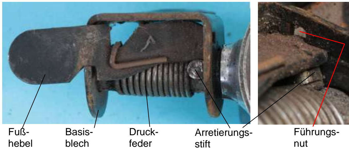
Bild 3.42: Kippvorrichtung ohne Abdeckung
