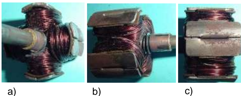
Bild 2.2: Sternanker: a) Lagerbuchse auf der Welle, b) Axialspielausgleichsfeder, c) Polschuh aus zwei Blechen
