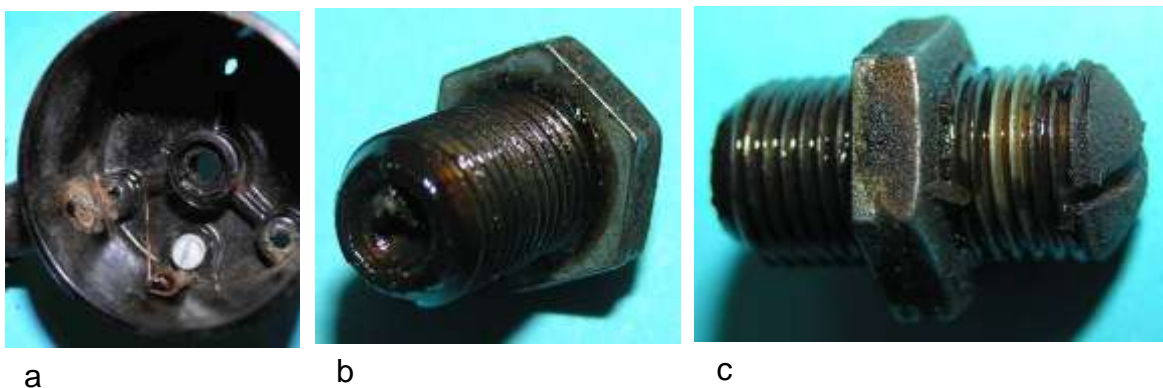
Bild 5.15: Einstellschraube des Axiallagers: a) Gehäusetopf mit zentraler Gewindebohrung, b) Sitz der Kugel, c) Schlitzschraube und Kontermutter
