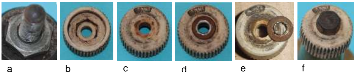
Bild 3.17: Reibradbefestigung: a) Untere Kontermutter, b) Kontur in der Reibradkeramik, c) Obere Seite des Reibrades, d) Eingelegte Passscheibe, e) Passscheibe f) Obere Kontermutter
