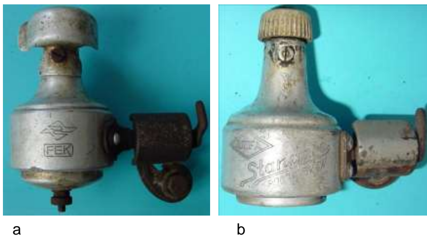
Bild 4.45: Vergleich: a) FEK-FLM 6 / 3B, 1960 b) AUFA-Standard 8007.1, 1958
