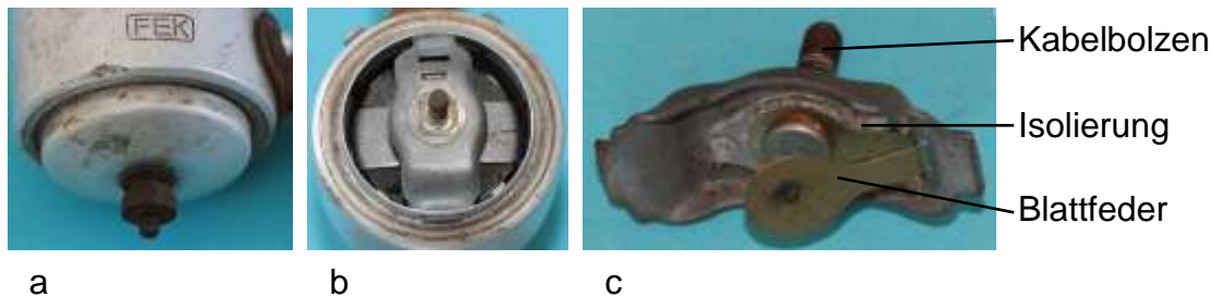
Bild 4.36: Bodenbereich: a) Montierter Boden, b) Im Zwischenring eingeklinkter Kontaktsteg, c) Federkontakt mit Kabelbolzen im Kontaktsteg
