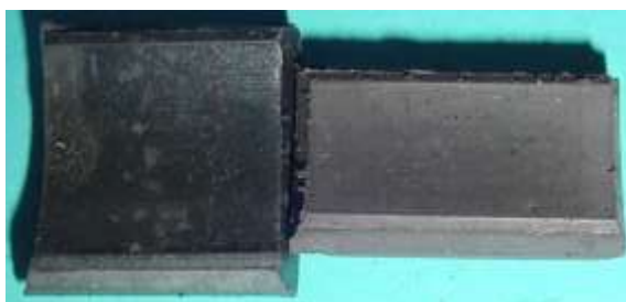
Bild 2.8: Blockmagnete: a) Kunststoff gebundener Magnet für einen vierpoligen Dynamo b) Keramikmagnet für einen achtpoligen Dynamo
