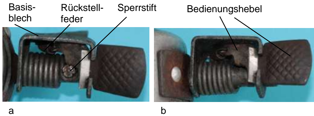
Bild 5.33: Einzelteile der Kippvorrichtung: a) Ruhestellung, b) Betriebsstellung
