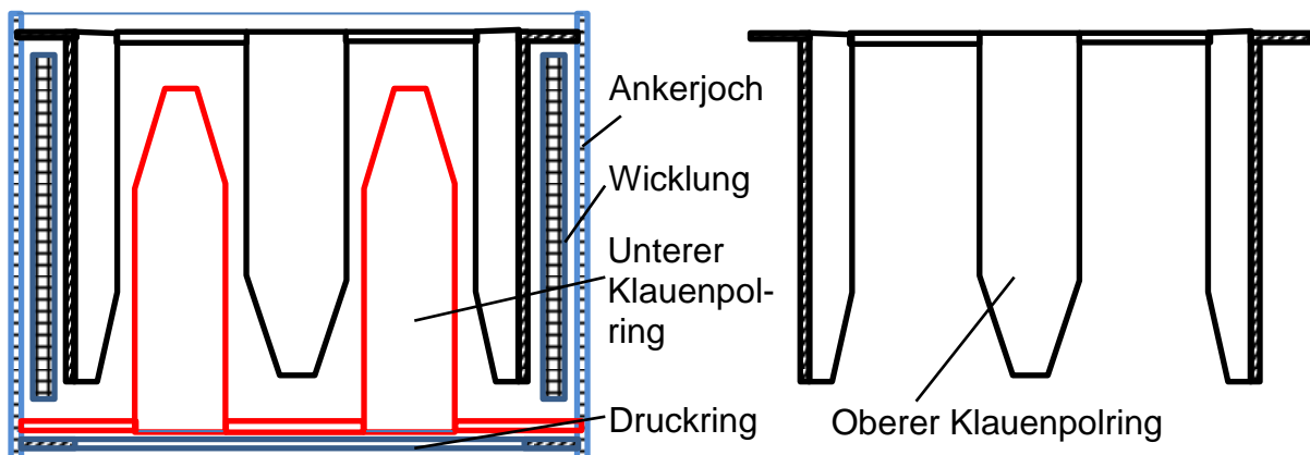
Bild 5.27: Prinzipskizze des vierteiligen Ankereisens
