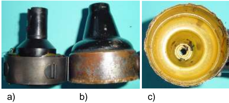
Bild 3.56: Gehäuse und Duroplastkonstruktion: a) Innerer Lagerhals mit Anker, b) Außenansicht des Gehäuses ohne Boden, c) Innenansicht des Lagerhalstopfes
