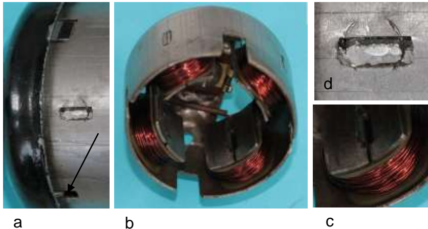
Bild 3.33: Magnetischer Kreis:
