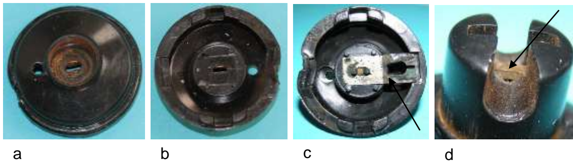
Bild 5.72: Boden: a) Unterseite, b) Innenseite, c) Schneidkontaktblech, d) Kabelanschlussblech
