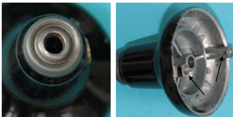
Bild 3.31: Lagerhals aus Zinkdruckguss a) Öldepot am oberen Lagerhalsrand b) Lagerhals mit Gewindebohrungen
