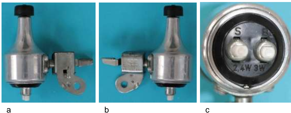
Bild 5.83: Typ 8007.9: a) und b) Seitenansichten, c) Bodenansicht
