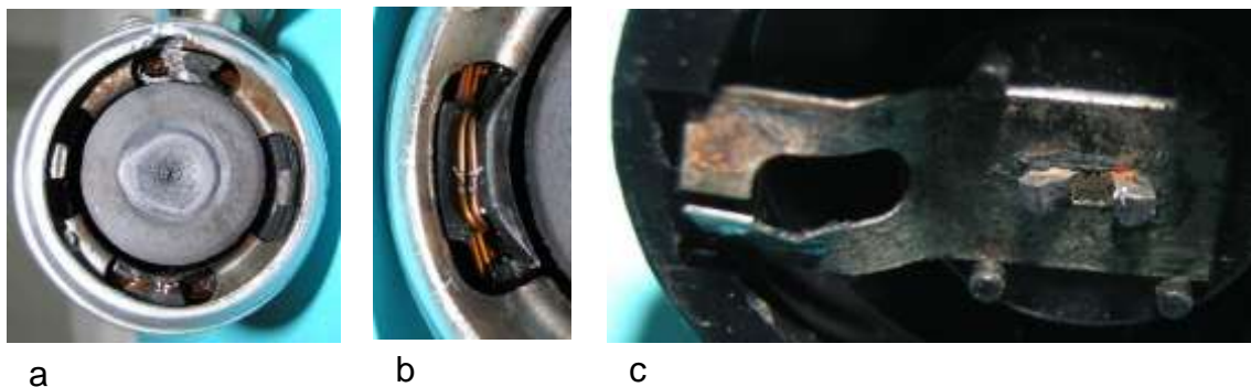
Bild 5.70: Kontaktierung: a) Entfernter Boden, b) Kontaktstützpunkt, c) Am Kabelkontaktblech befestigte Schneidklemme
