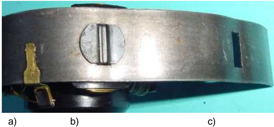
Bild 3.62: AbgeboGENES Ständerjoch: a) Massekontakt, b) Abgewinkelte Befestigungslaschen c) Ausnehmung für einen Polschaff
