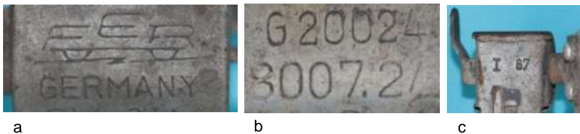
Bild 5.50: Beschriftung der Dynamo-Lampen-Kombination 8007.2: a) Firmenlogo und Produktionsstandort, b) Prüfzeichen G 20024, c) Fertigungsdatum I 67
