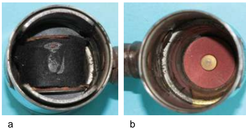
Bild 3.21: Gehäusetopf: a) Eingebauter Anker b) Isoliert eingesetzter Kabelanschlussbolzen
