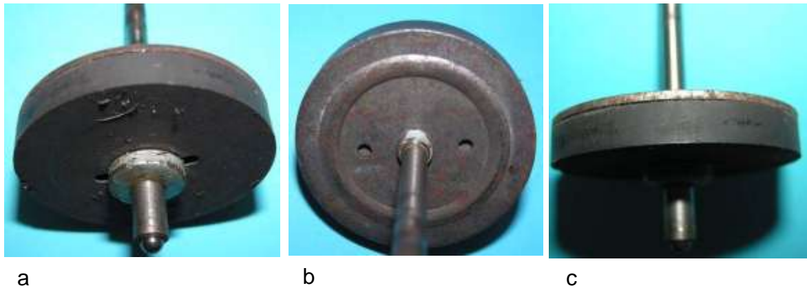
Bild 5.12: Welle und Polrad: a) Bund unterhalb des Magneten, b) Verschraubung des Jochs mit der Welle, c) Mantelfläche des Polrades
