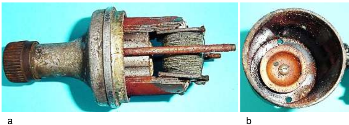
Bild 2.2: Bauteile des Dynamos: a) Lagerhals mit den Generatorelemente, b) Innenraum des Gehäusetopfes
