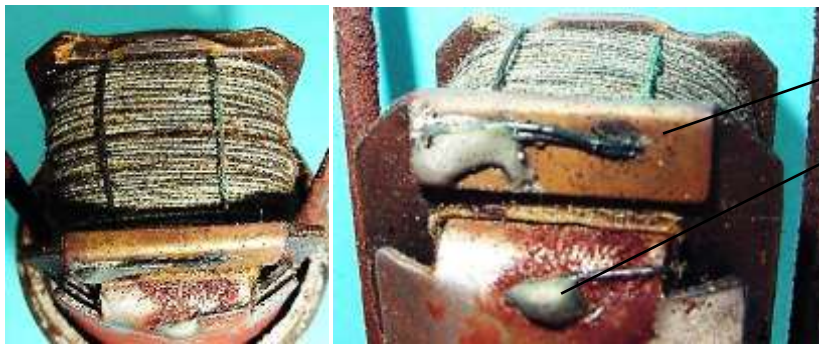
Bild 2.6: Kontakte des Ankers
