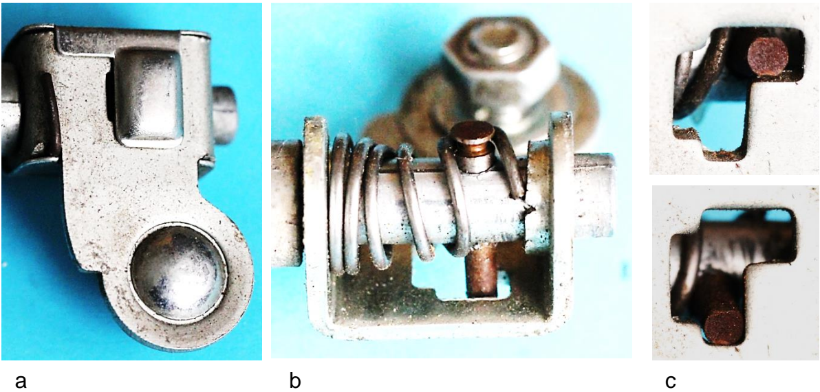
Bild 12.80: Kippvorrichtung: a) Verdeckte Winkelkulissee auf der Rückseite, b) Drehbolzen, Sperrstift und Druckfeder, c) Positionen des Sperrstifts in der Winkelkulissee
