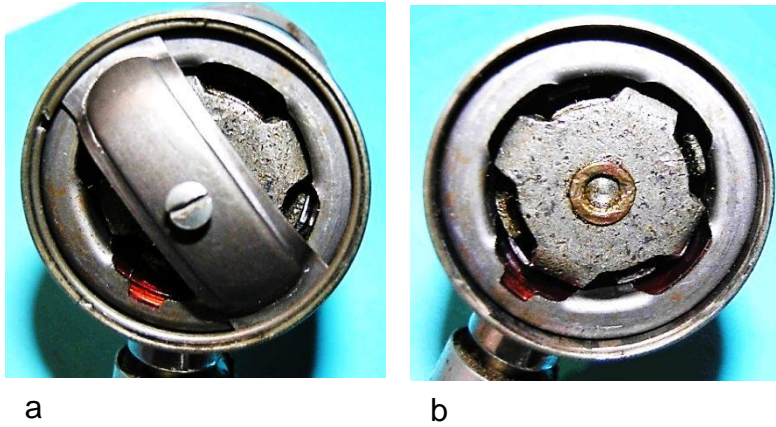
Bild 12.33: Abgenommener Boden: a) Steg mit Bodenschraube, b) Stirnseiten des Polrades und des Ankers
