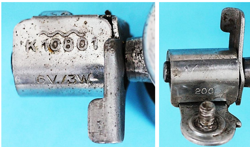
Bild 12.59: Einprägungen auf dem Abdeckblech
