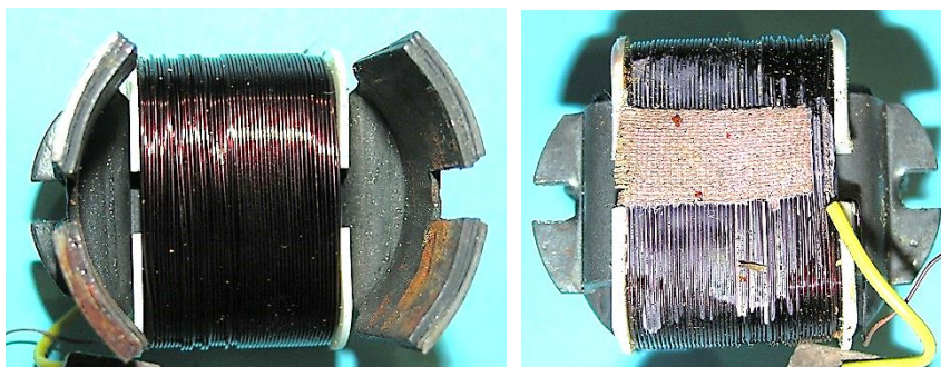
Bild 12.13: Obere und untere Ankerspulen-seite
