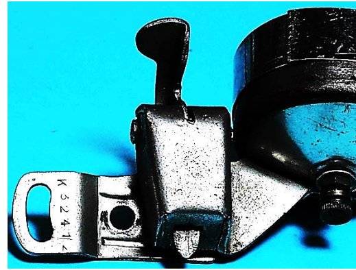
Bild 12.29: Kippschalterprinzip: a) Boden mit Kabelanschlussbolzen und angenietetem Flansch der Kippvorrichtung, b) Kippvorrichtung mit der K-Nummer K 32412
