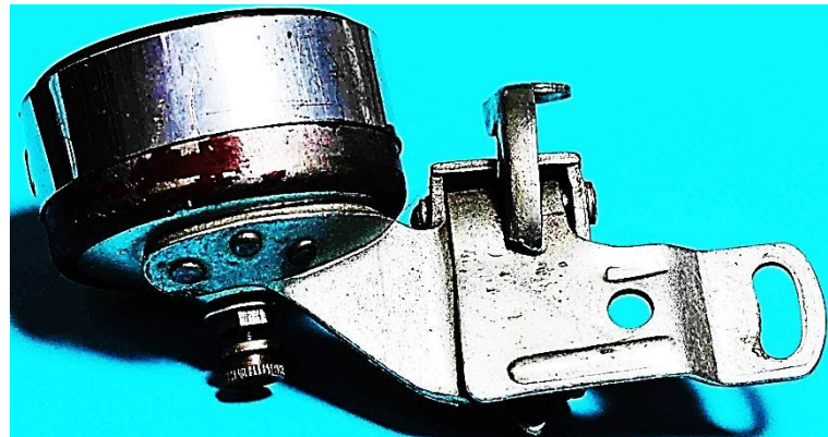
Bild 12.30: Baugruppen: a) Achtpoliges Klauenpolrad mit zweipoligem Magneten. b) Gehäusetopf mit der Kippvorrichtung
