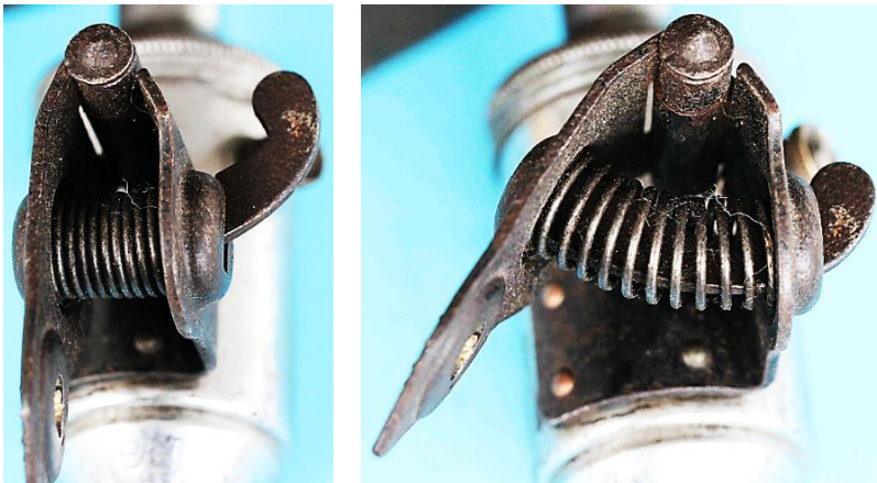
Bild 2.1: Berko-Kippvorrichtung
