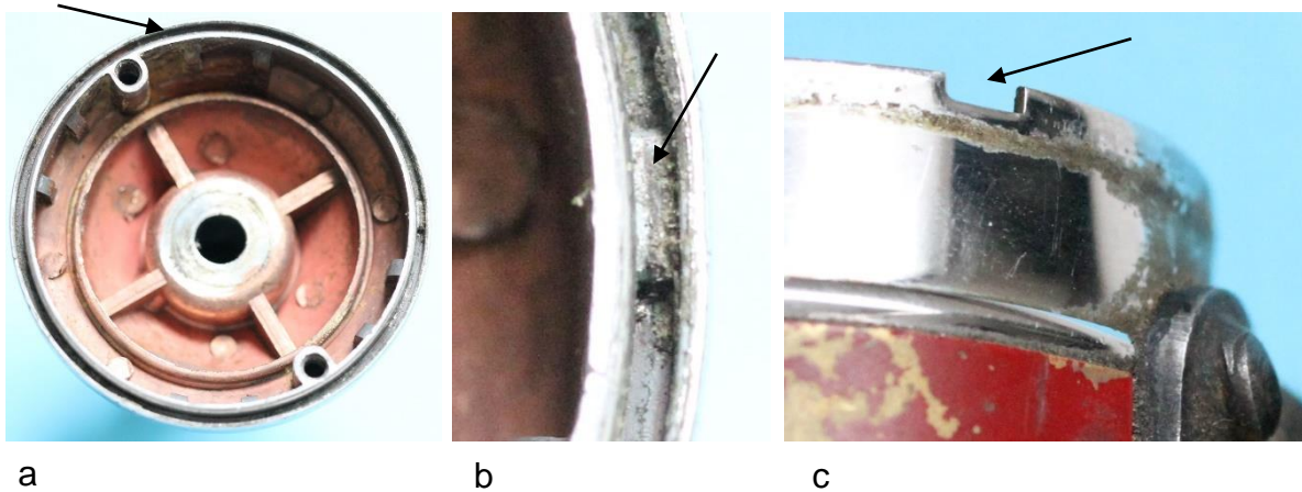
Bild 12.2: Wasserdichte Einpassung des Gehäusetopfes im Lagerhalsfuß: a) 2 mm tiefe Rille im Lagerhalsfuß, b) Zapfen in der Rille, c) Ausnehmung im Gehäuse
