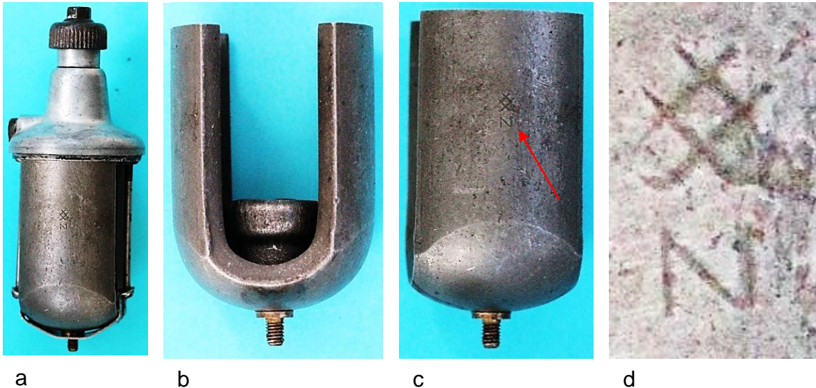
Bild 7.15: Tulpenmagnet: a) Lagerhals mit angeschraubtem Gehäusekopf, b) Spurlager im Magnetjoch, c) Magnetschenkel mit Firmenstempel, d) Firmenstempel
