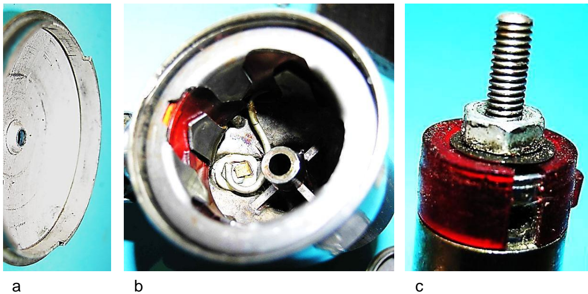
Bild 12.35: Baugruppen: a) Boden, b) Anker, c) Öllochabdeckung
