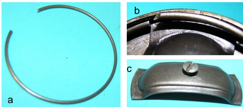
Bild 12.34: Montageteile a) Drahtfeder b) Eingelegter Drahtfeder- ring c) Montagesteg
