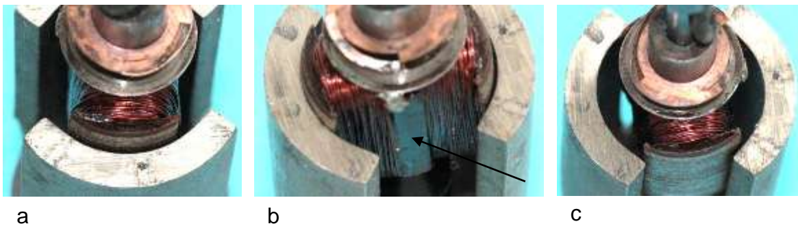
Bild 2.9: Vergleich der Polbreiten: a) Polbreiten verhalten sich wie 2:3, b) Gegenüberstellung der Polrücken, c) Ankerpolbreite entspricht etwa der Breite der Polrücke des Magneten
