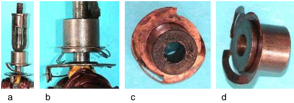
Bild 2.13: Massekontakt: a) Massekontakt mit den Lagern auf der Welle, b) Massekontakt zwischen Anker und unterm Lager, c) und d) Sitz der Federbürste auf dem unteren Lager
