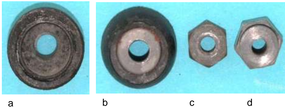
Bild 2.6: Kabelanschluss: a) Am Gehäuse anliegende Fläche des Isolierteils, b) Mit einer Scheibe verstärkte Seite, c) Mutter zur Befestigung des Isolierteils, d) Mutter zum Anklemmen des Kabelschuhs
