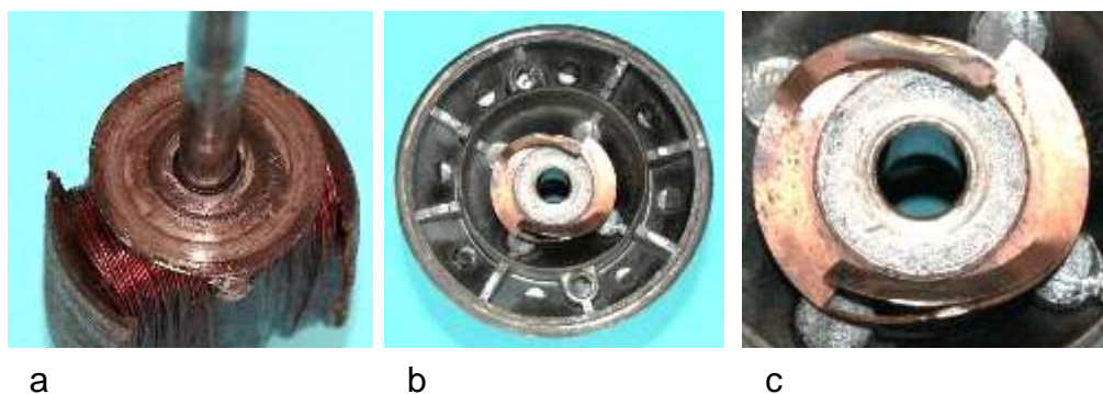
Bild 2.12: Massekontakt: a) Masseschleifscheibe, b) Lagerhals mit Massebürste, c) Massebürste mit unterem Gleitlager
