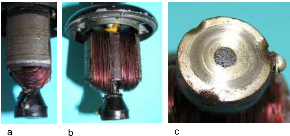
Bild 2.10: Anker (29 Bleche, 0,7 mm stark, Durchmesser 28 mm): a) Polfläche, b) Polrücke mit Zwischensteg, c) Spannungsführende Schleifscheibe
