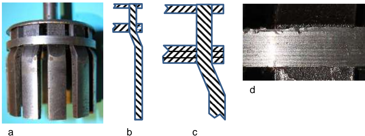
Bild 4.9: Fixierung der Magnete im Joch: a) Polrad, b) und c) Schnitte durch einen Pol, d) Überdrehte Oberfläche des unteren Jochs
