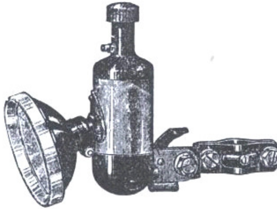
Bild 1.5: Melas-Nonox mit angebaute Lampe 2,1 W für Rennmaschinen
