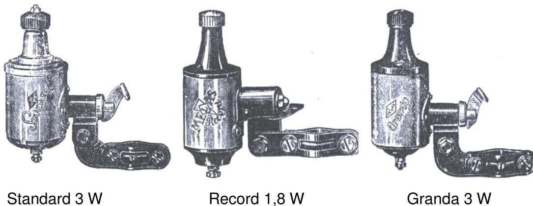
Bild 1.4: Stab-Magnet-Dynamos ????
